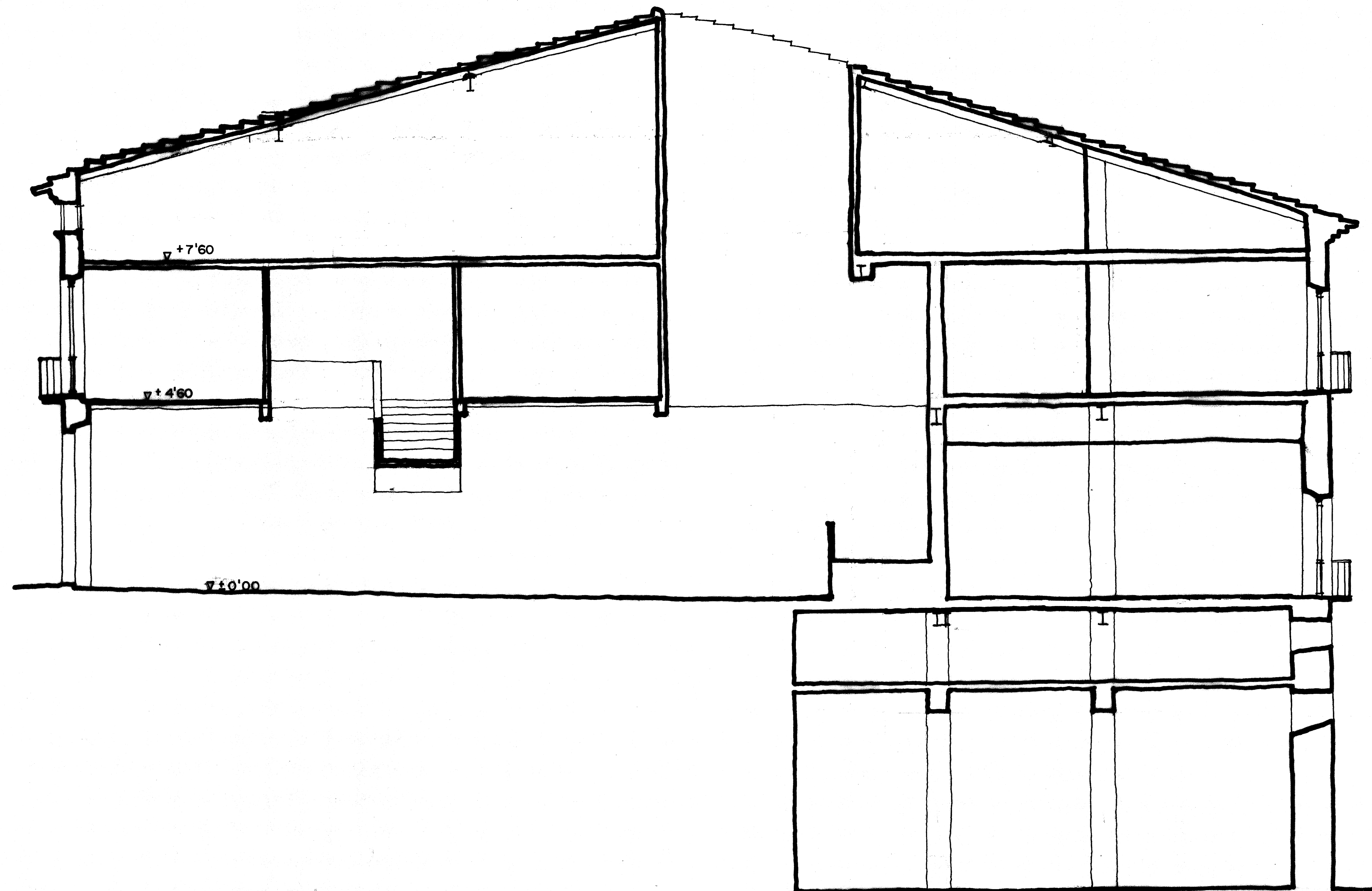
SECCION
