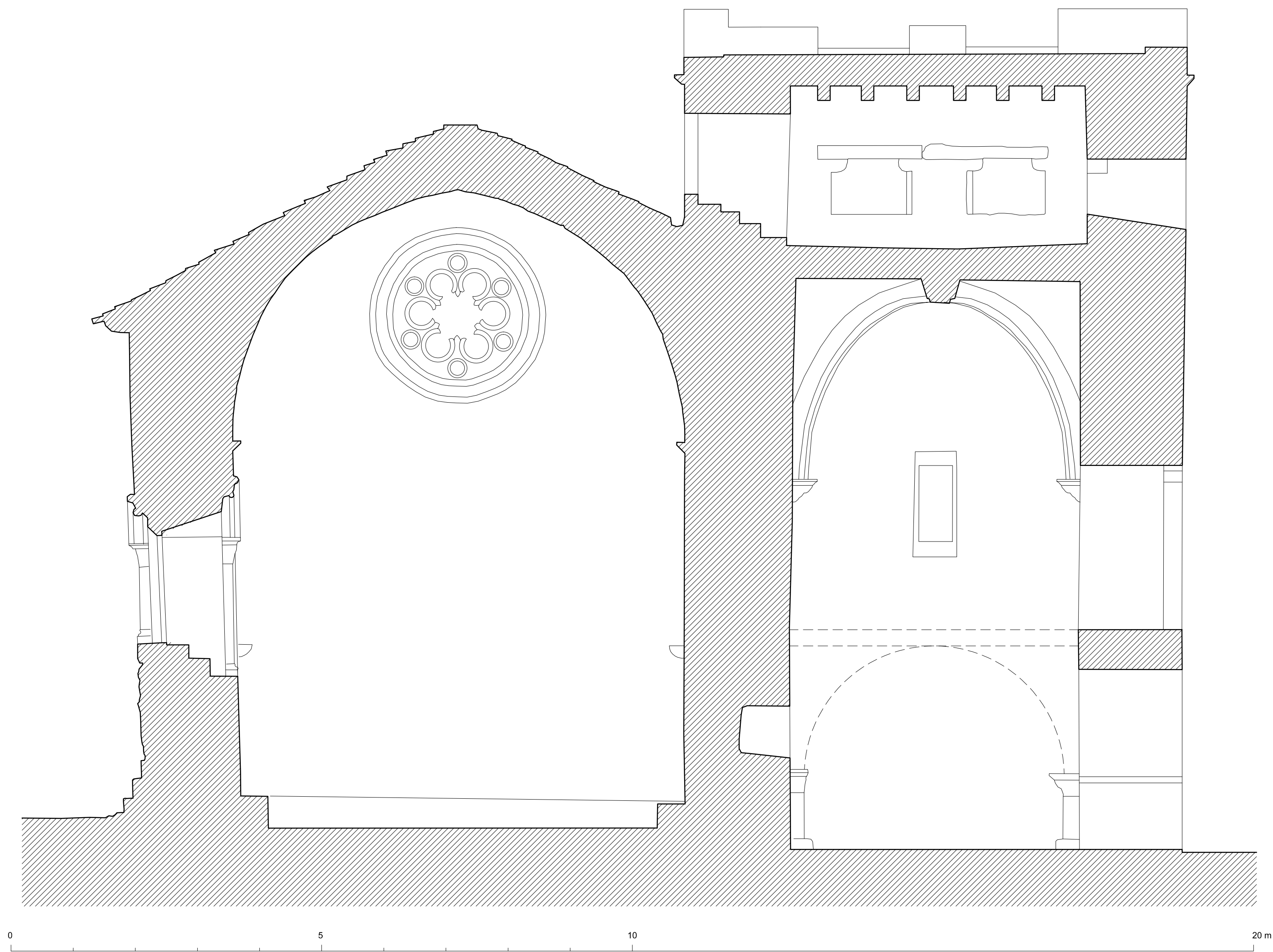
IGLESIA SANJUANISTA DE SAN MIGUEL ARCANGEL. CIZUR MENOR. NAVARRA. Seccion transversal por la torre
