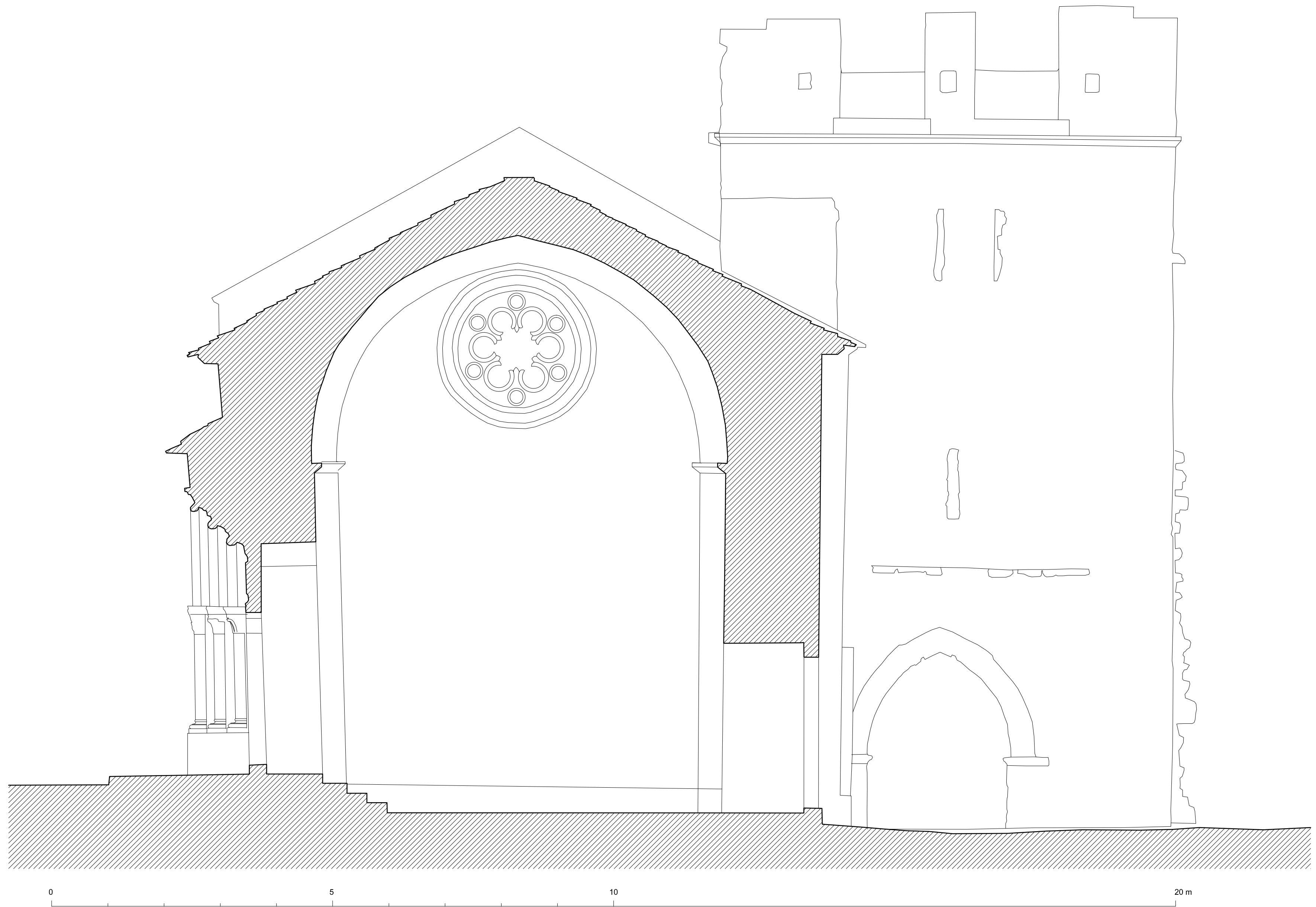
IGLESIA SANJUANISTA DE SAN MIGUEL ARCANGEL. CIZUR MENOR. NAVARRA. Seccion transversal
