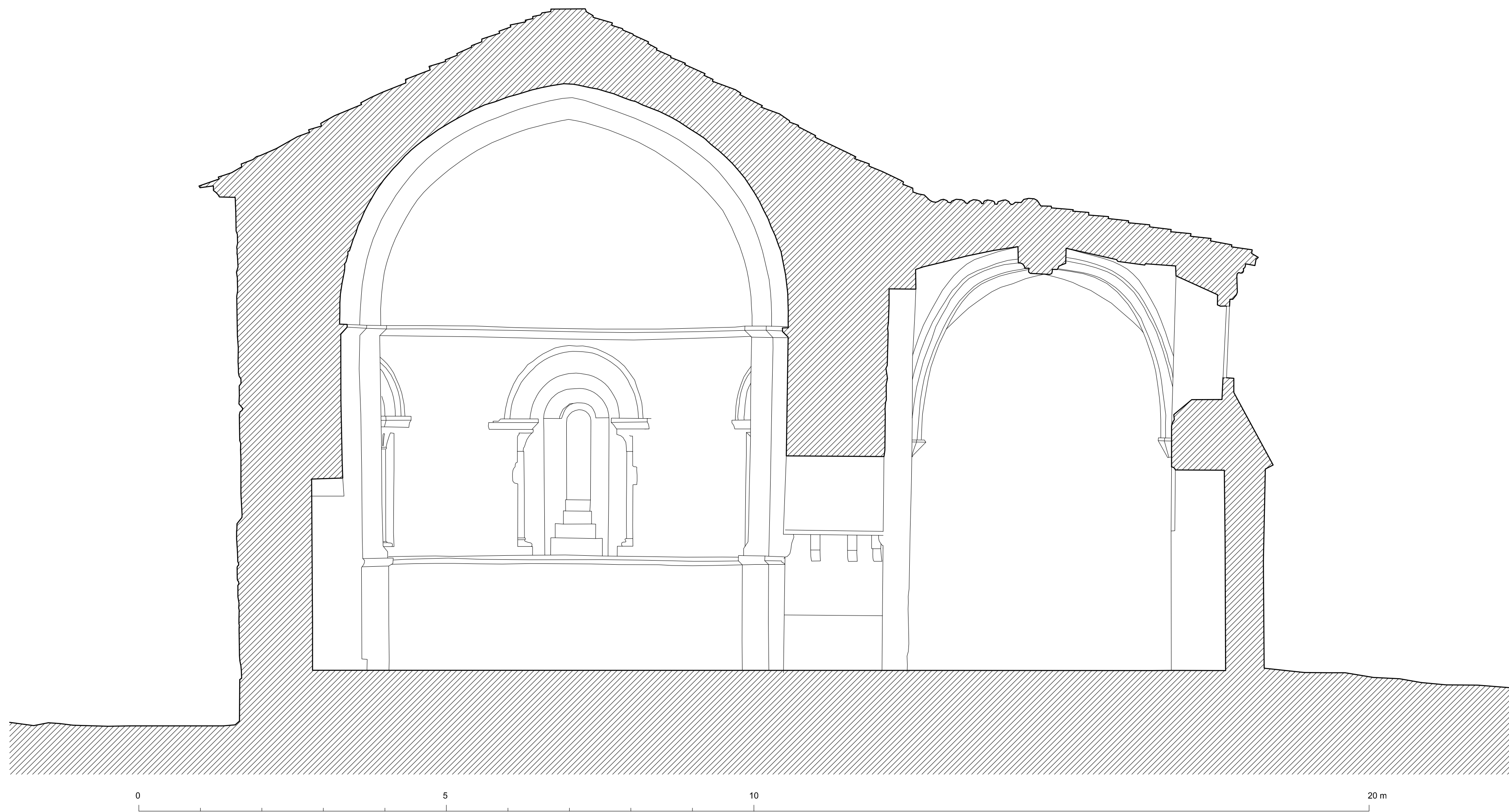
IGLESIA SANJUANISTA DE SAN MIGUEL ARCANGEL. CIZUR MENOR. NAVARRA. Sección transversal cabecera
