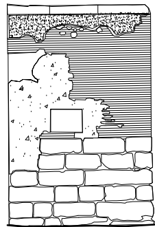
ALZADO B
