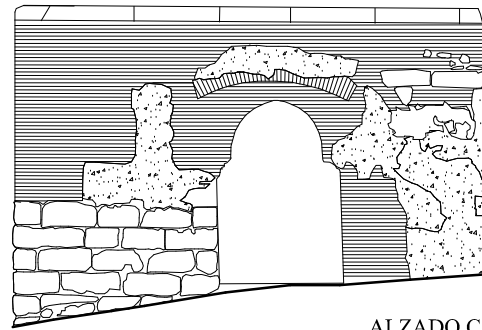
ALZADO C
