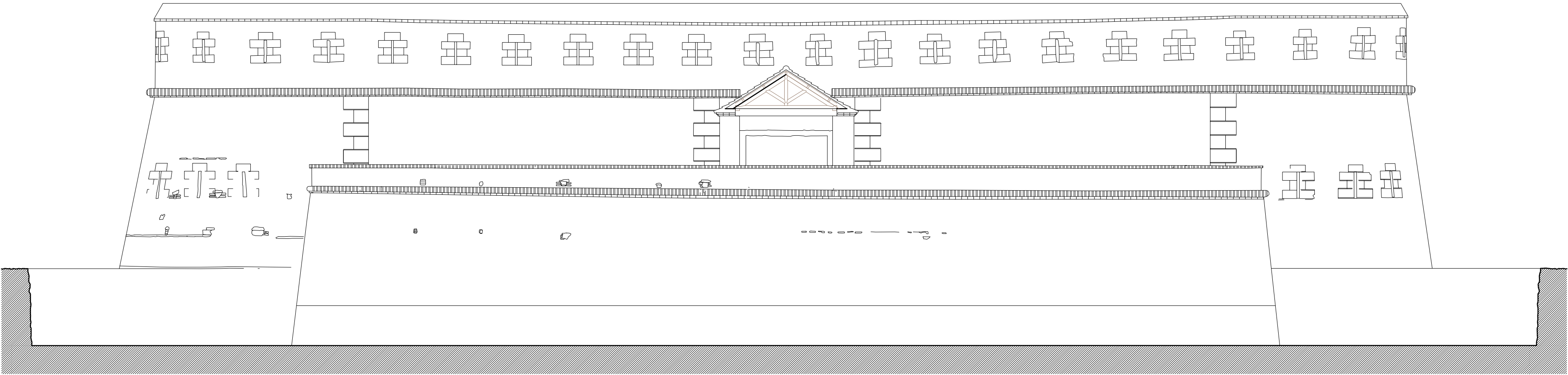
ALZADO SUR
