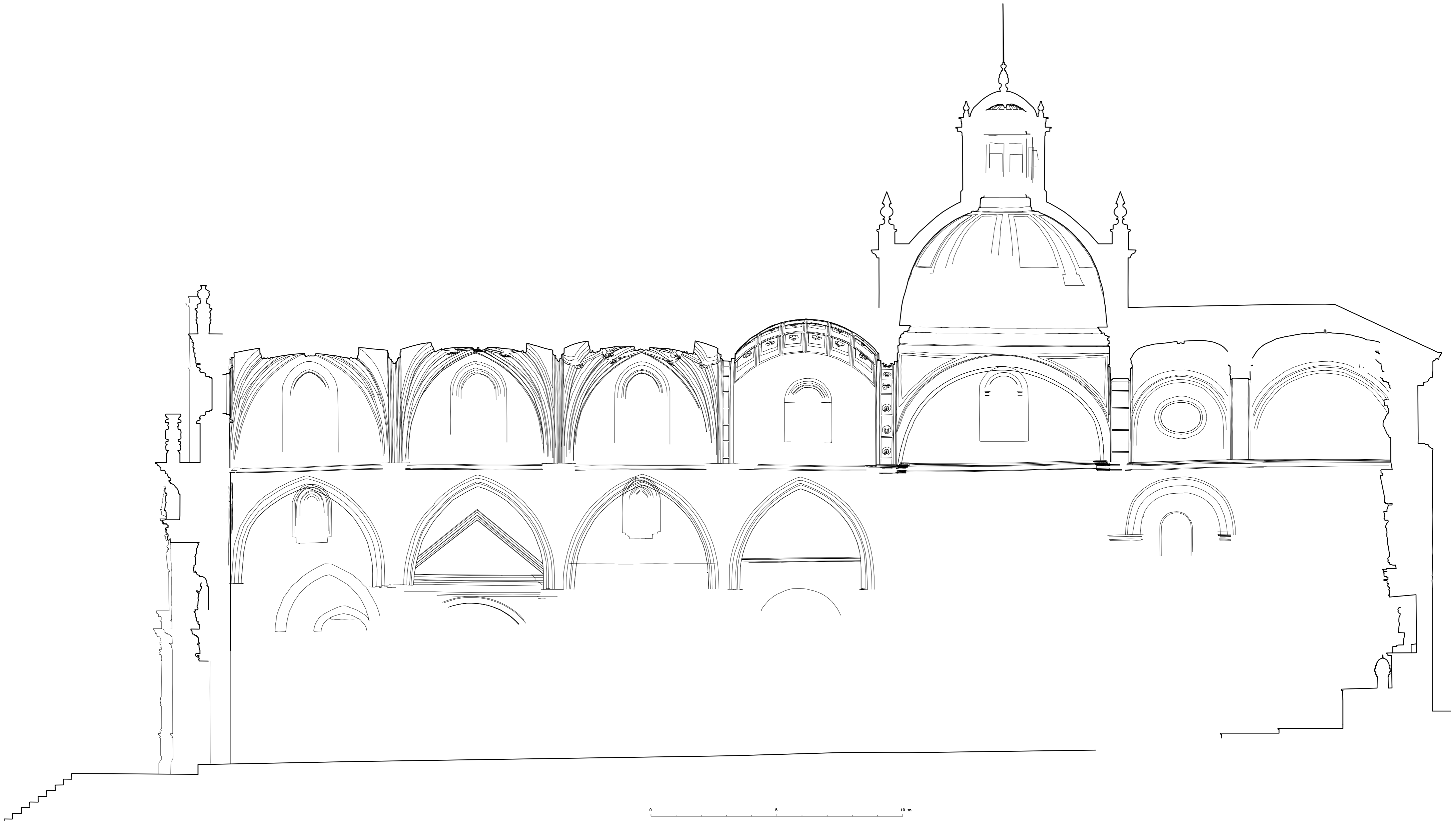
0 5 10 m IGLESIA PARROQUIAL DE SAN MIGUEL. MORON DE LA FRONTERA (SEVILLA) ESCUELA DE ESTUDIOS ARABES. CSIC. A. Almagro / arq. I. Zúñiga / arq. tec.
