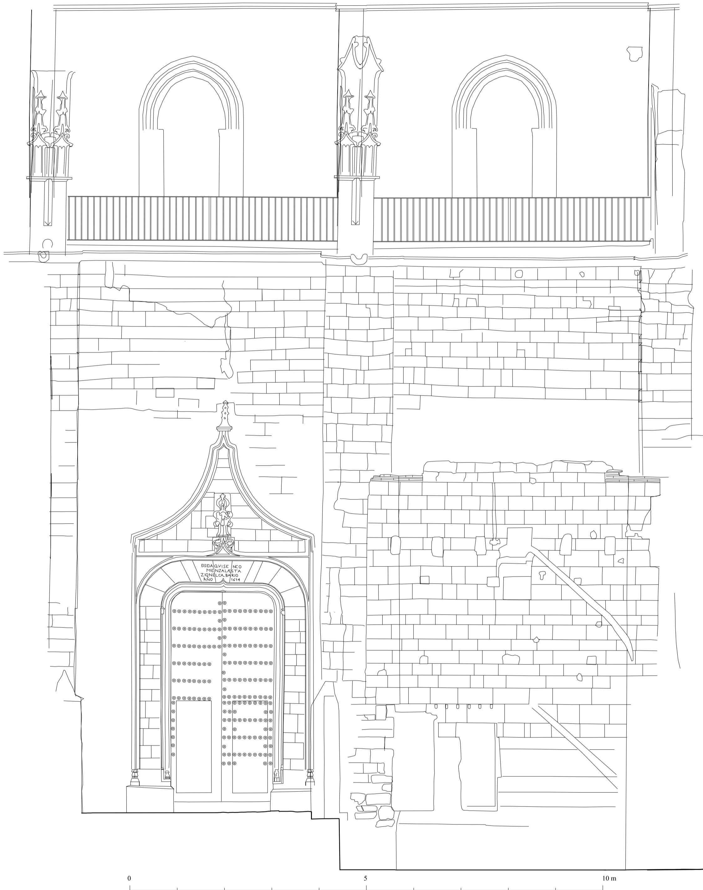
IGLESIA PARROQUIAL DE SAN MIGUEL. MORON DE LA FRONTERA (SEVILLA) ESCUELA DE ESTUDIOS ARABES. CSIC. A.Almagro arquitecto. PUERTA NORTE
