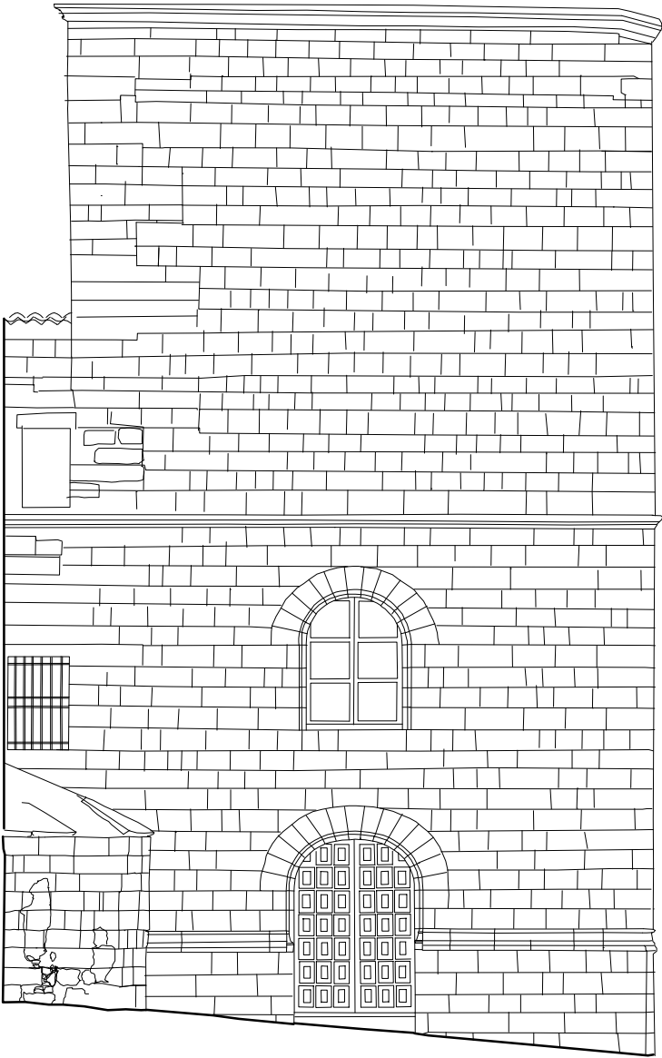
0 5 10 m CASAS CONSISTORIALES. BAEZA A. Almagro / arq. 1990
