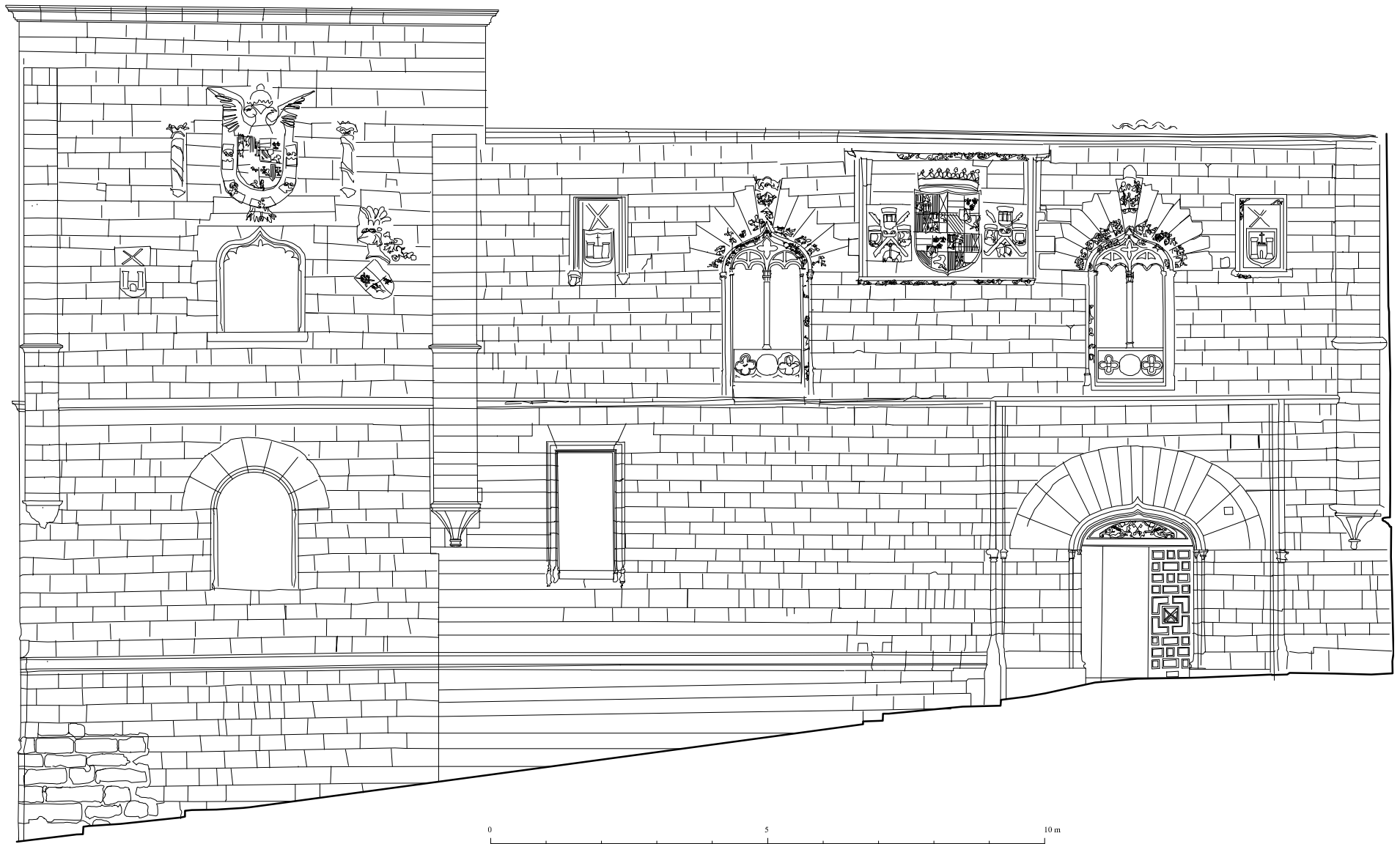
CASAS CONSISTORIALES. BAEZA A. Almagro / arq. 1990
