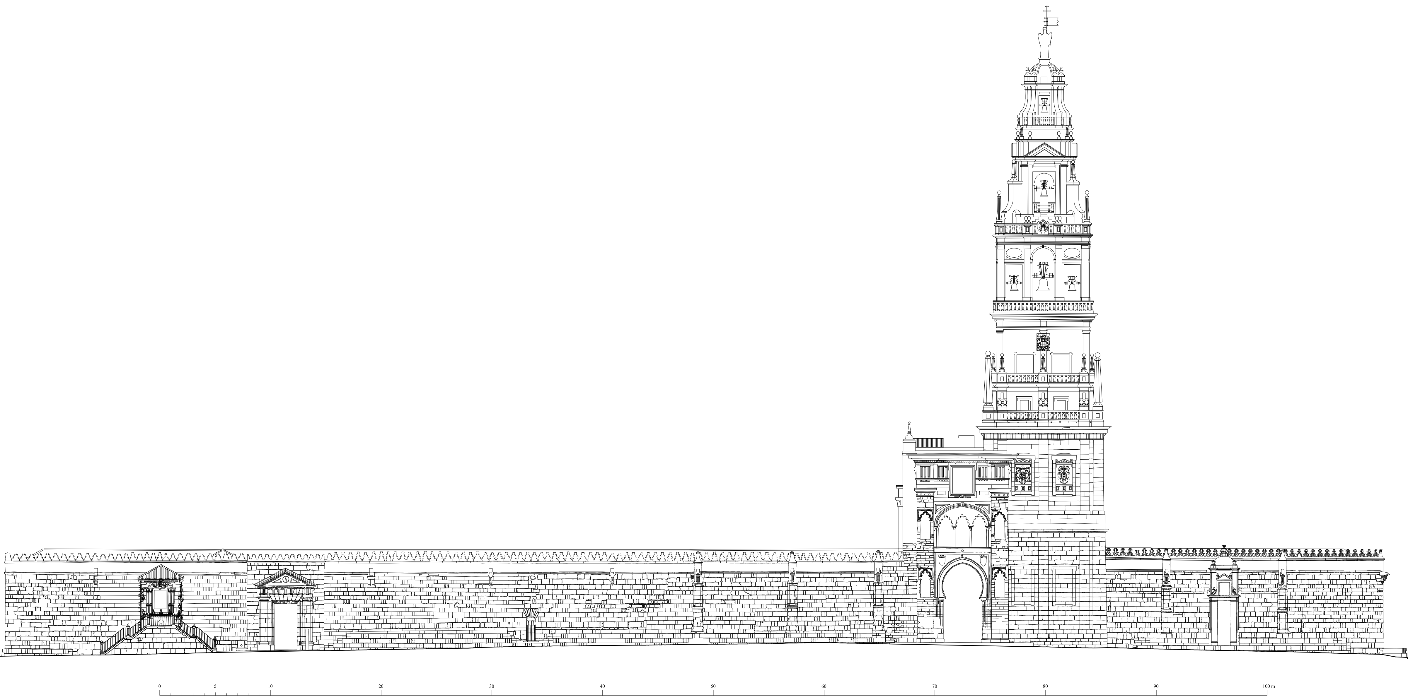
CATEDRAL EX-MEZQUITA DE CORDOBA. ALZADO NORTE.
