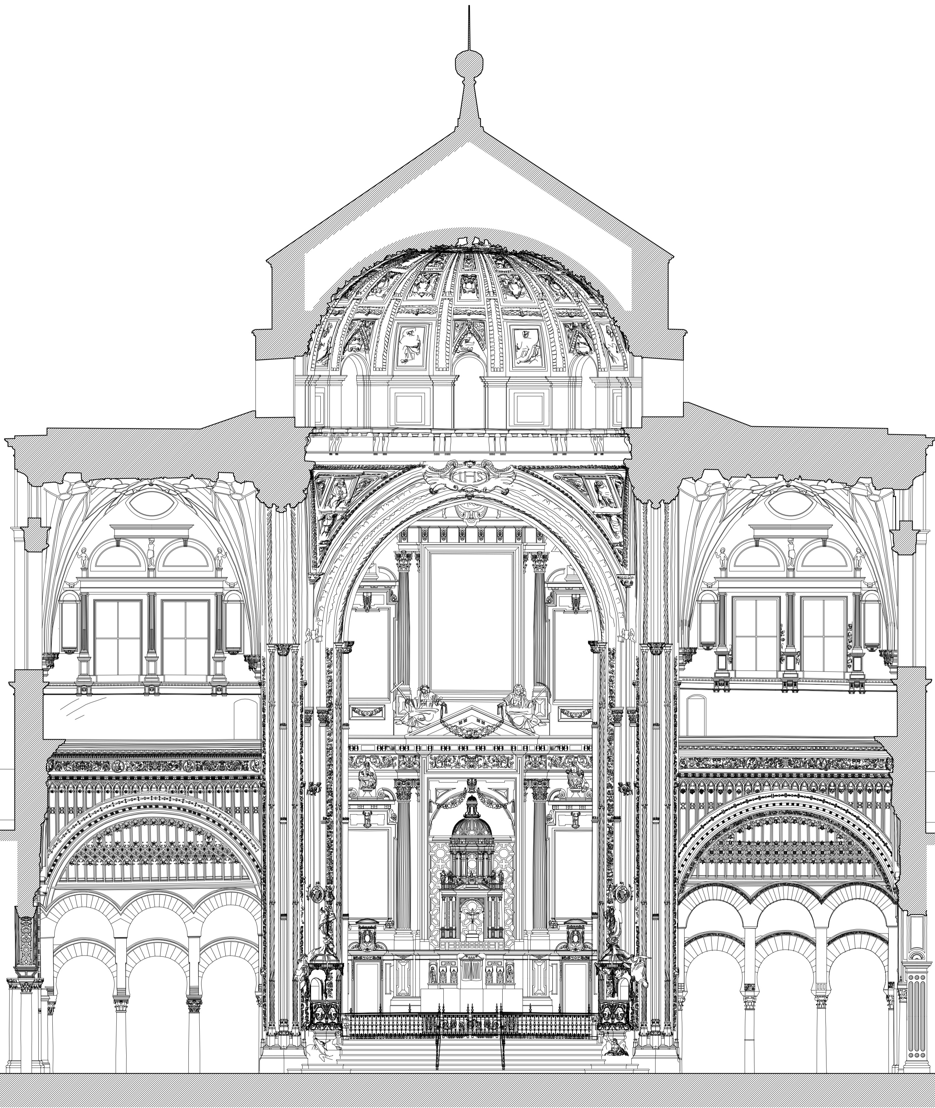
CATEDRAL DE CORDOBA. SECCION TRANSVERSAL DEL CRUCERO RENACENTISTA A.Almagro / arq. I. Zúñiga / arq. tec 1985-2020
