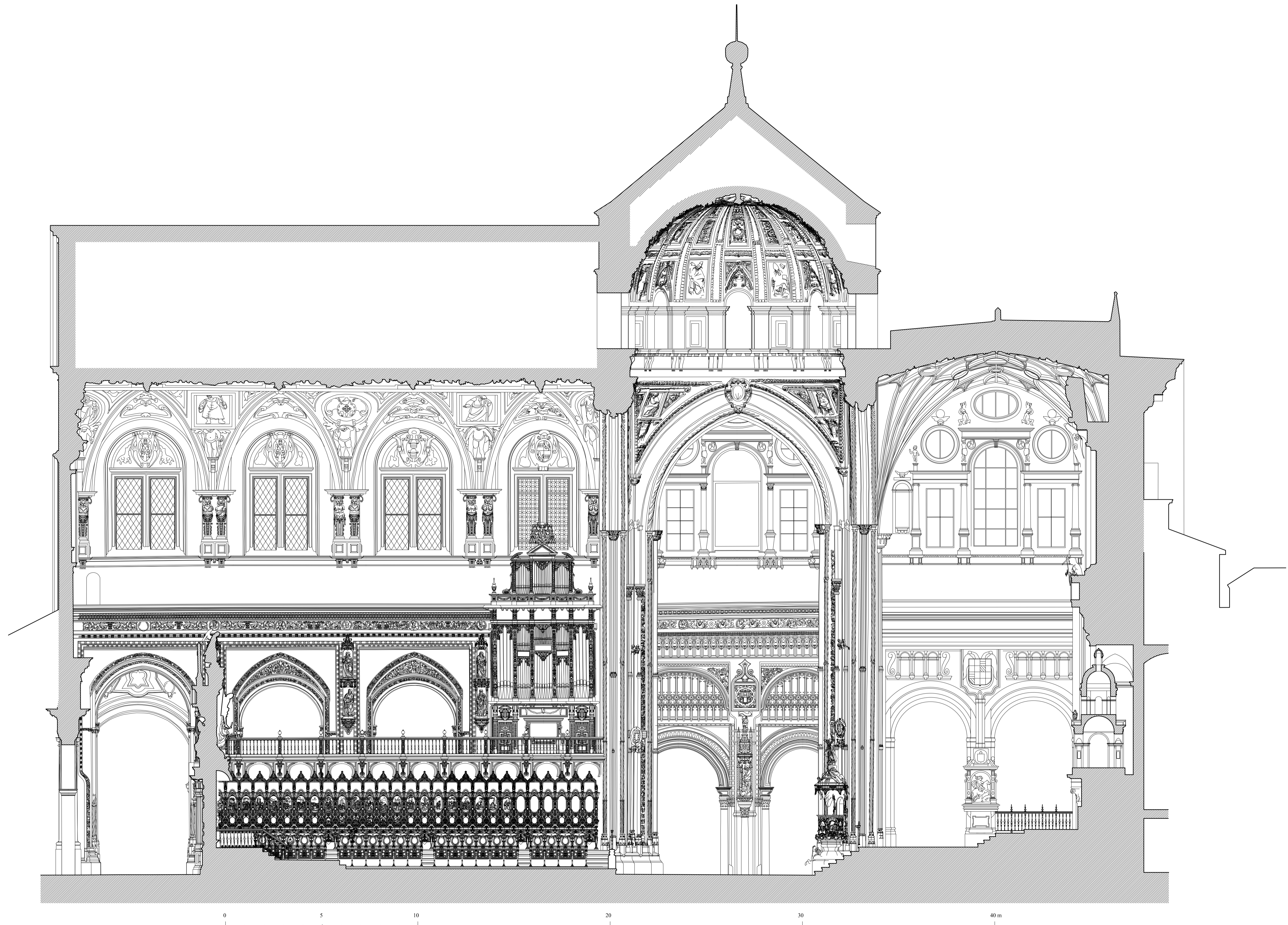
CATEDRAL DE CORDOBA. SECCION LONGITUDINAL DEL CRUCERO RENACENTISTA A. Almagro / arq. I. Zúñiga / arq. tec. 1985-2020
