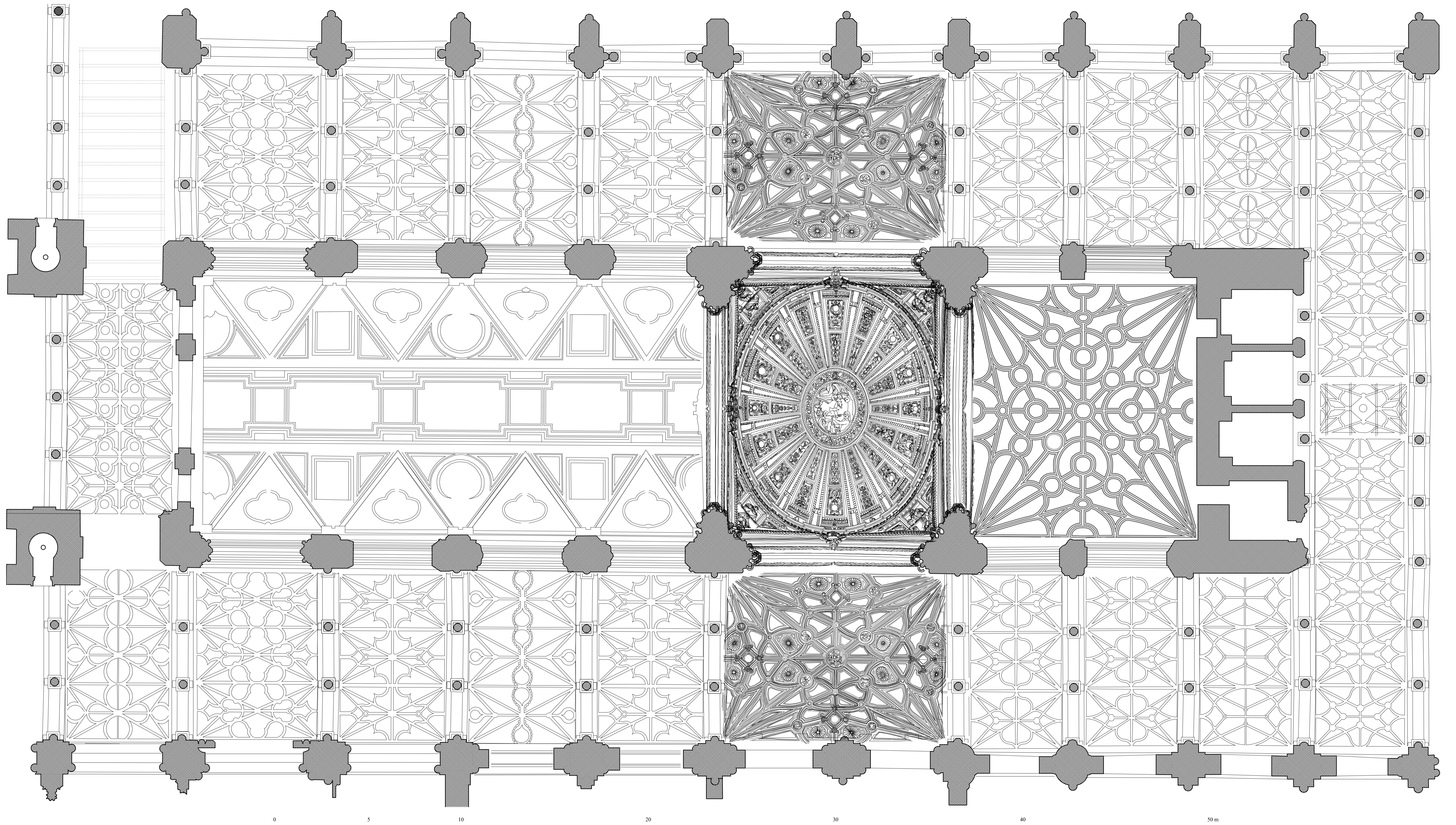
CATEDRAL DE CORDOBA. PLANTA DEL CRUCERO RENACENTISTA A.Almagro / arq. 1985-2020
