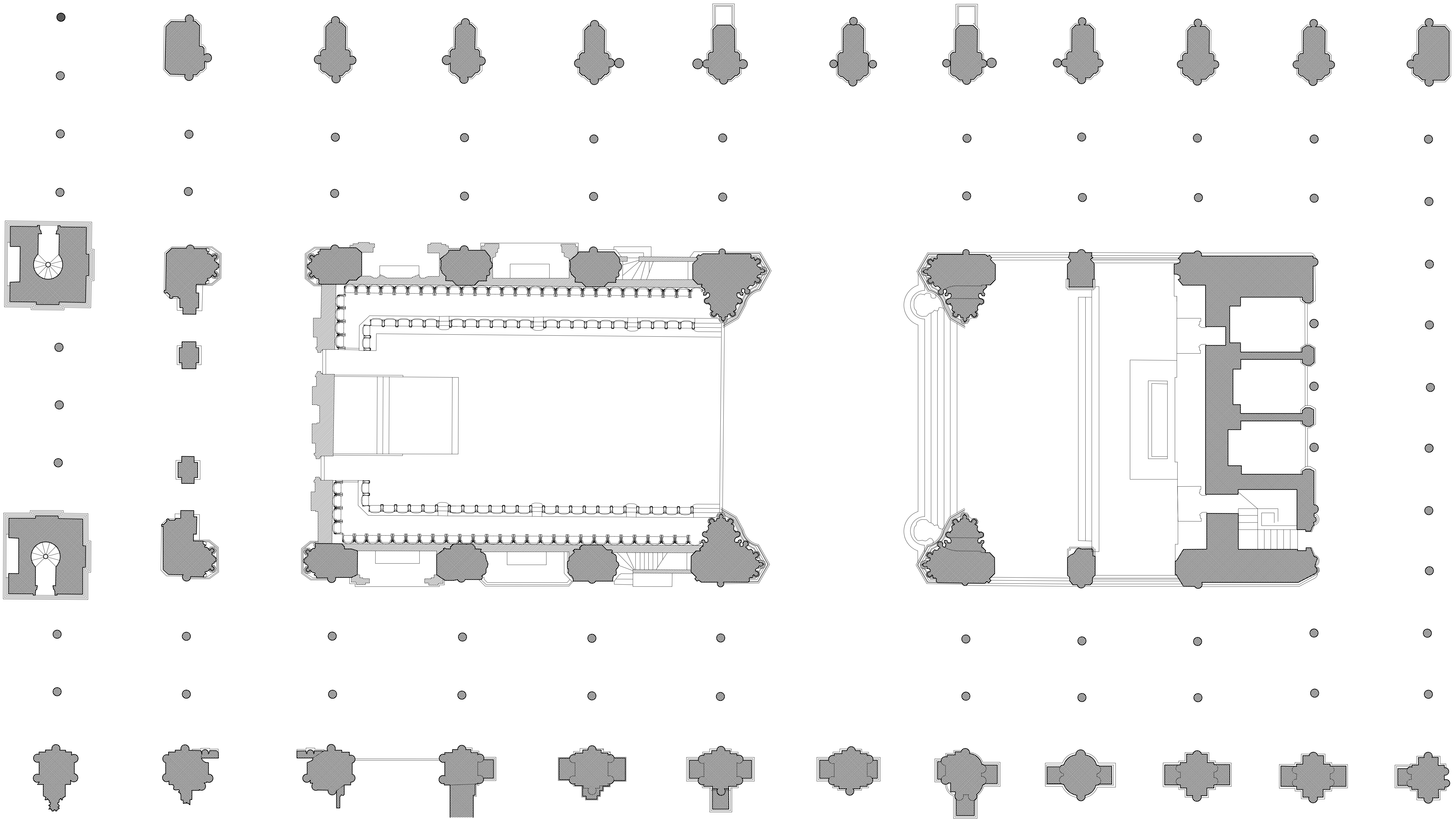
CATEDRAL DE CORDOBA. PLANTA DEL CRUCERO RENACENTISTA A.Almagro / arq. 1985-2020
