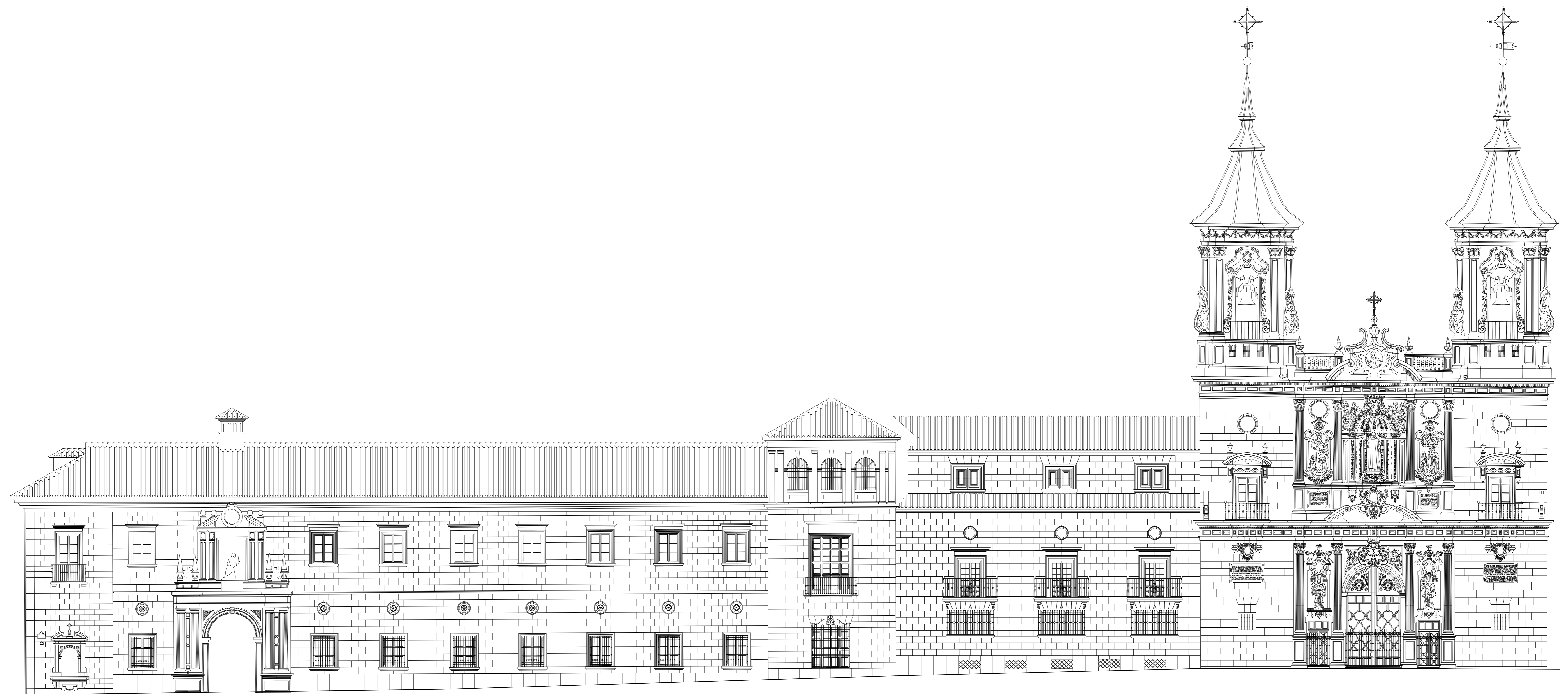
HOSPITAL DE SAN JUAN DE DIOS. GRANADA ALZADO PRINCIPAL Levantamiento realizado por el Prof. Antonio Arriaga Corles, los alumnos de la asignatura de Levantamiento de Edificios de la Escuela Técnica Superior de Arquitectura de Granada de los cursos 2006-2007 y 2007-2008 y la Escuela de Estudios Árabes del CSIC
