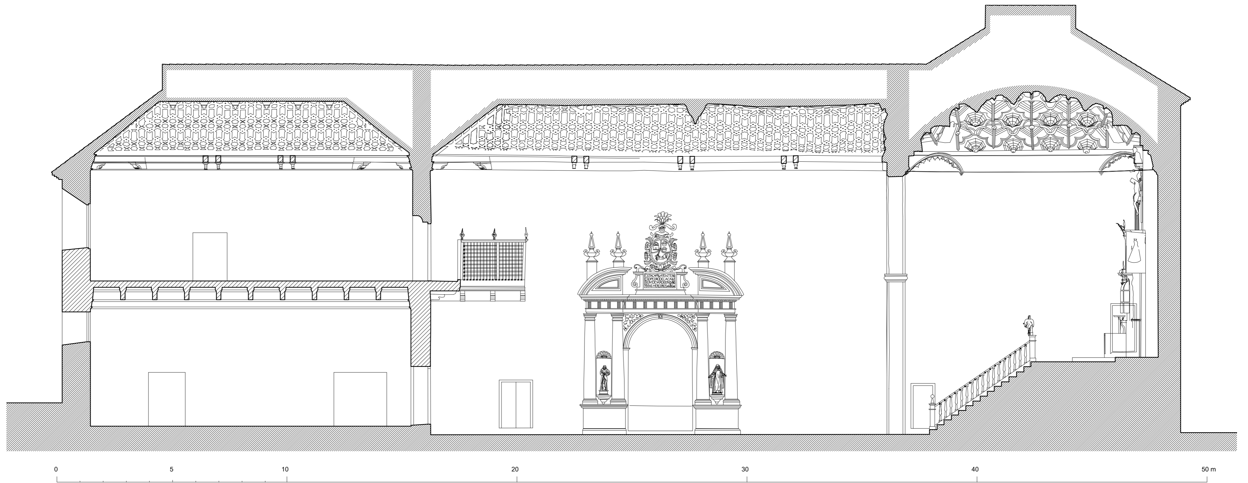
CONVENTO DE SANTA ISABEL LA REAL. GRANADA C. Sanchez, A. Almagro / arqs. 2009
