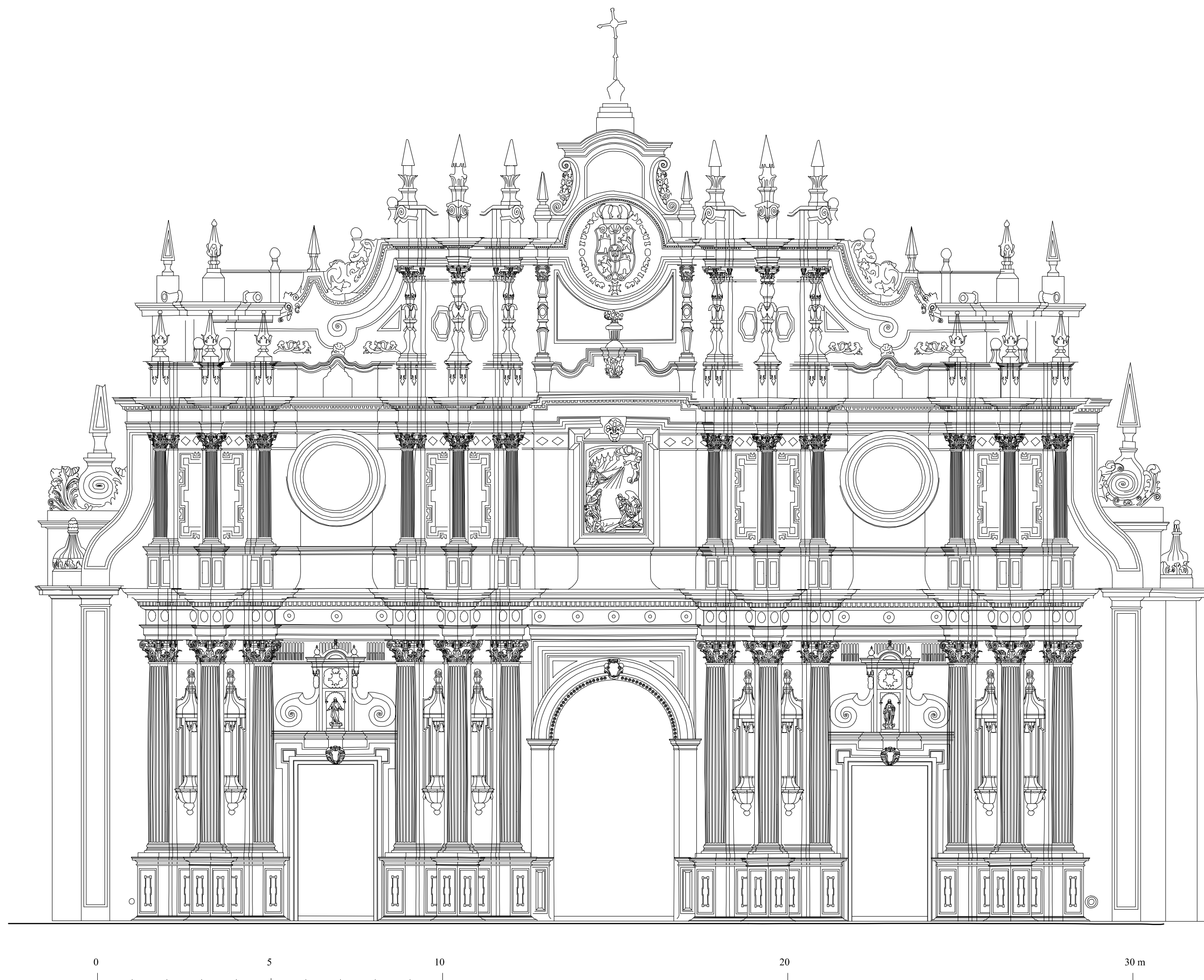
CATEDRAL DE GUADIX. ALZADO PRINCIPAL A. Almagro / arq. I. Zúñigas / arq.tec.
