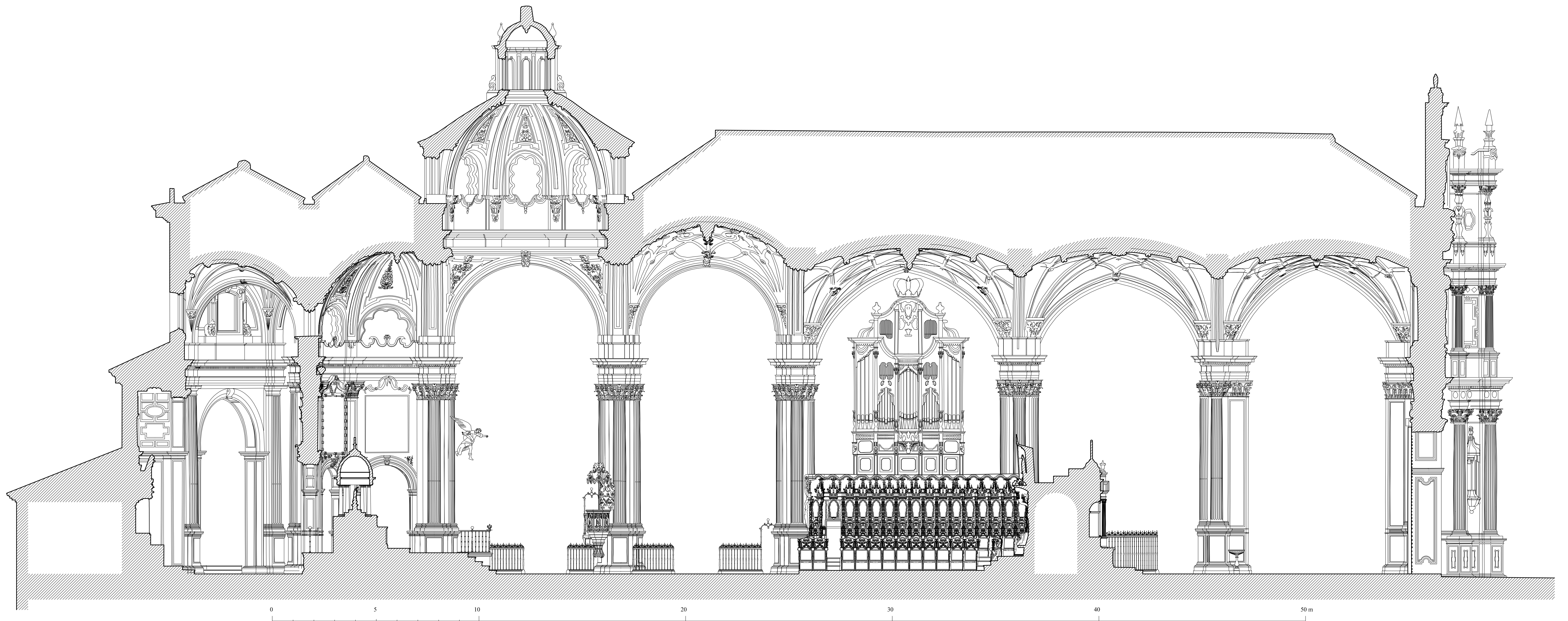
CATEDRAL DE GUADIX. SECCION LONGITUDINAL A. Almagro / arq. I. Zúñiga / arq.tec.
