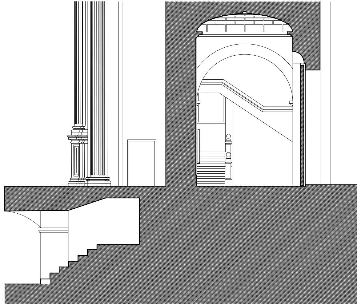
SECCION 1-1
