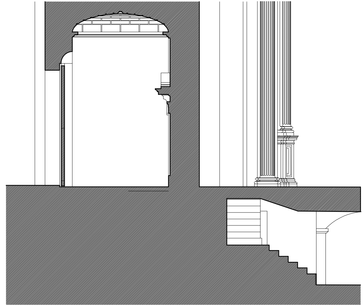
SECCION 2-2
