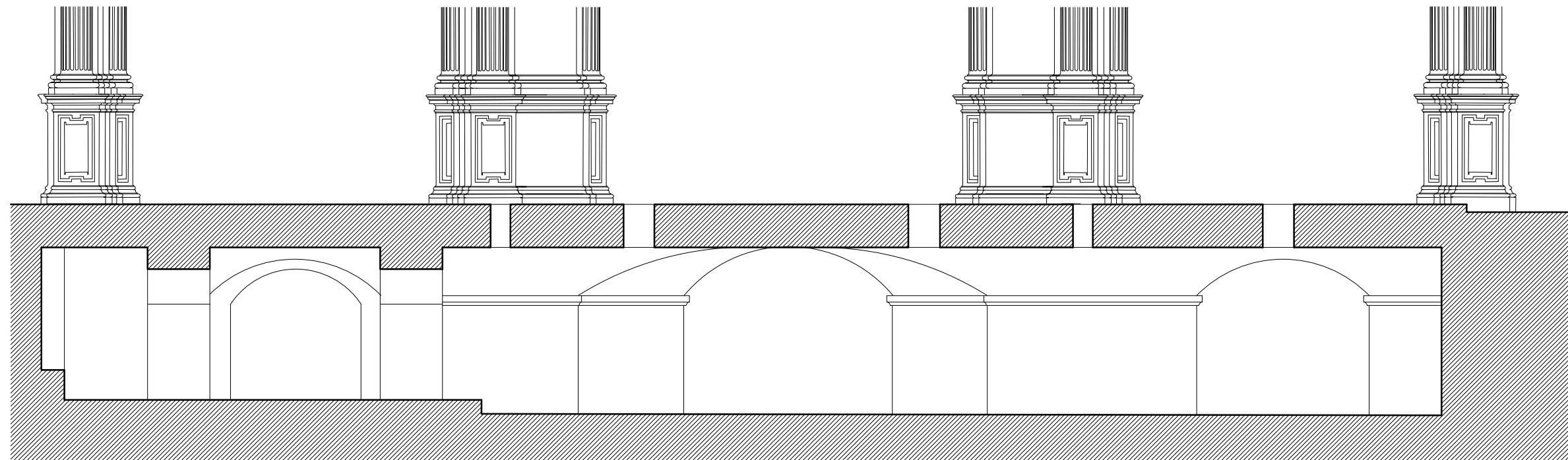
SECCION D-D
