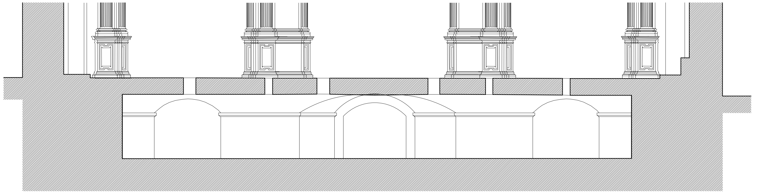
SECCION C-C
