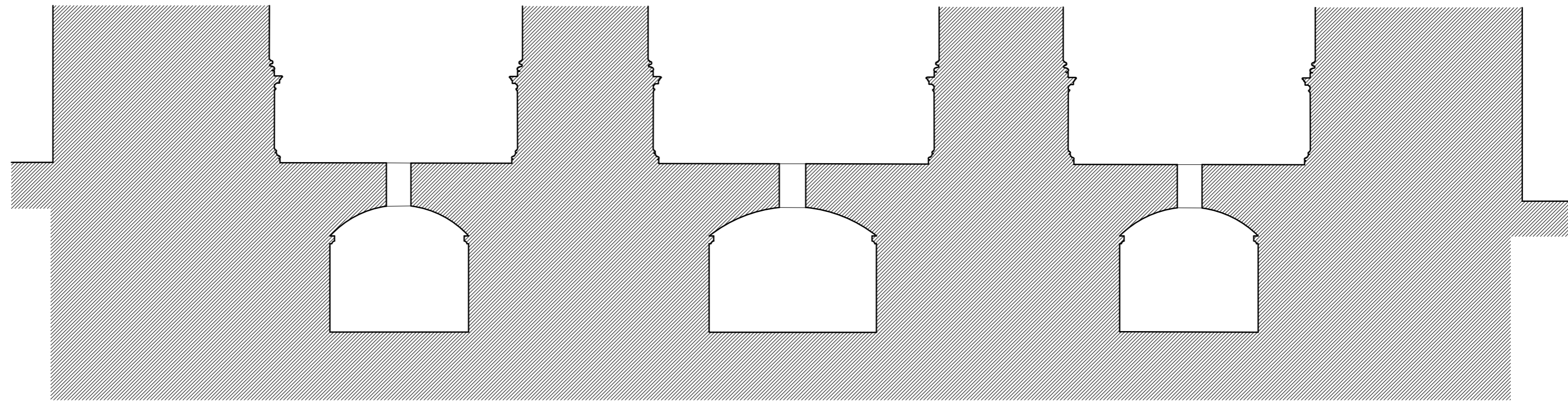
SECCION B-B
