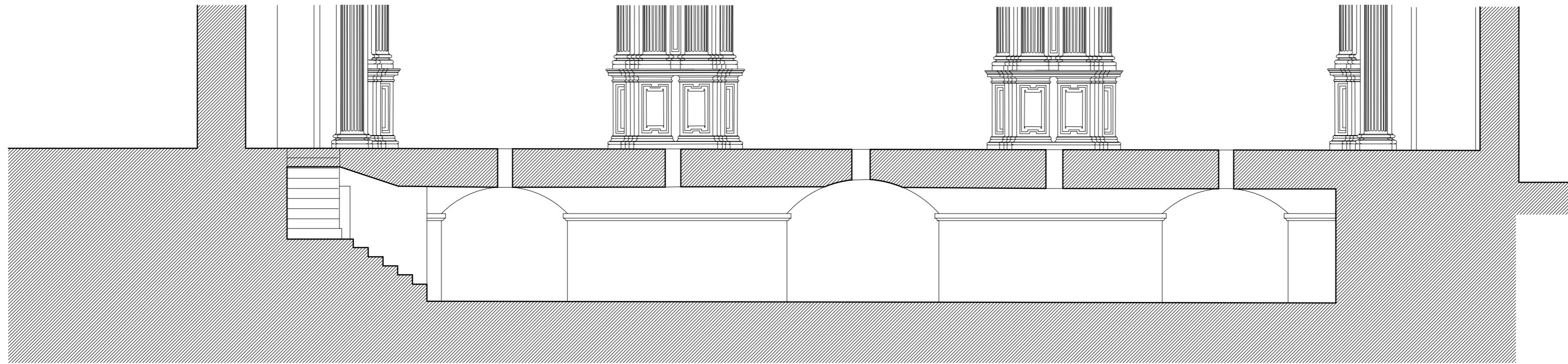
SECCION A-A
