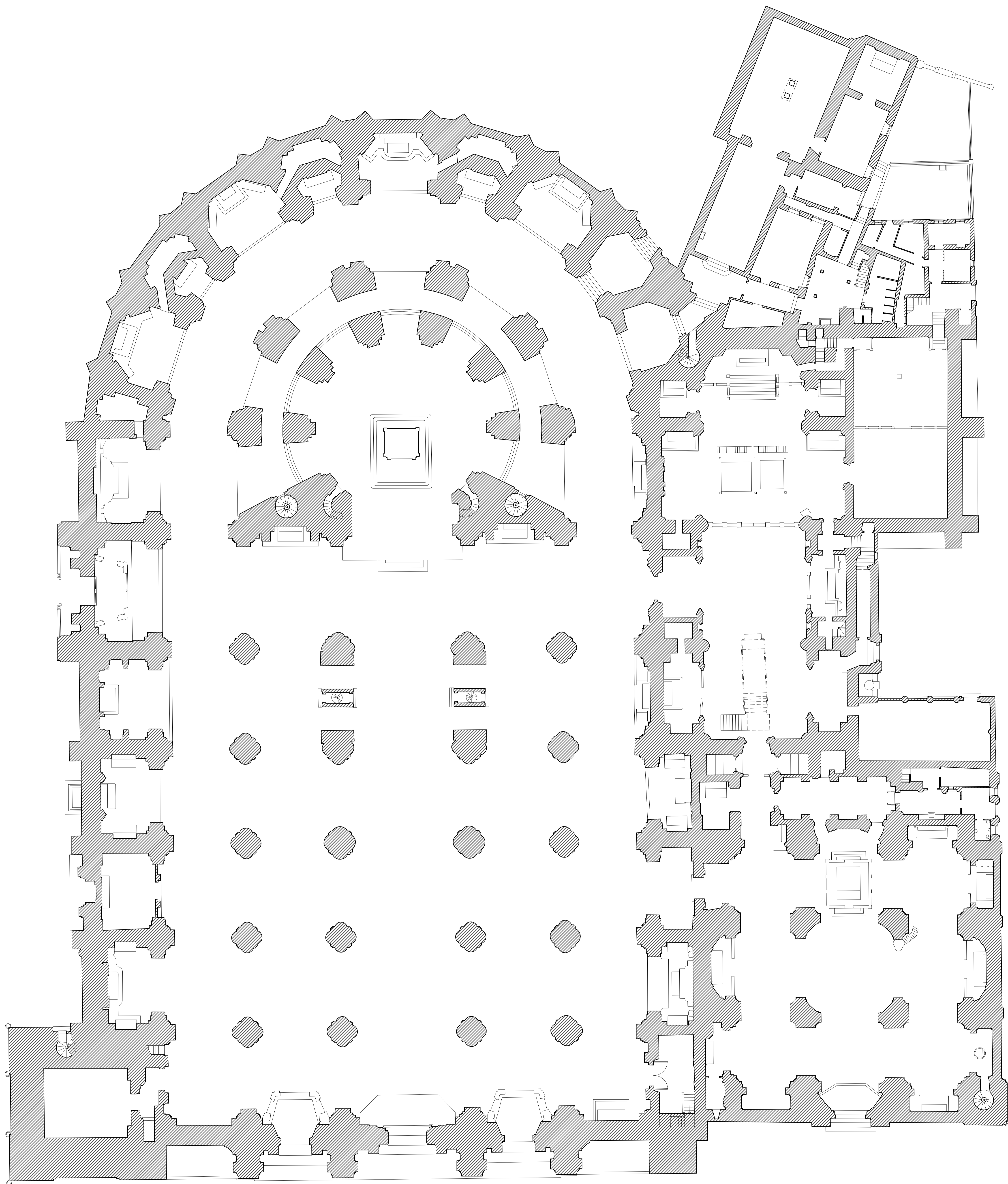
CATEDRAL DE GRANADA. PLANTA A. Almagro y J. A. Portillo y otros.
