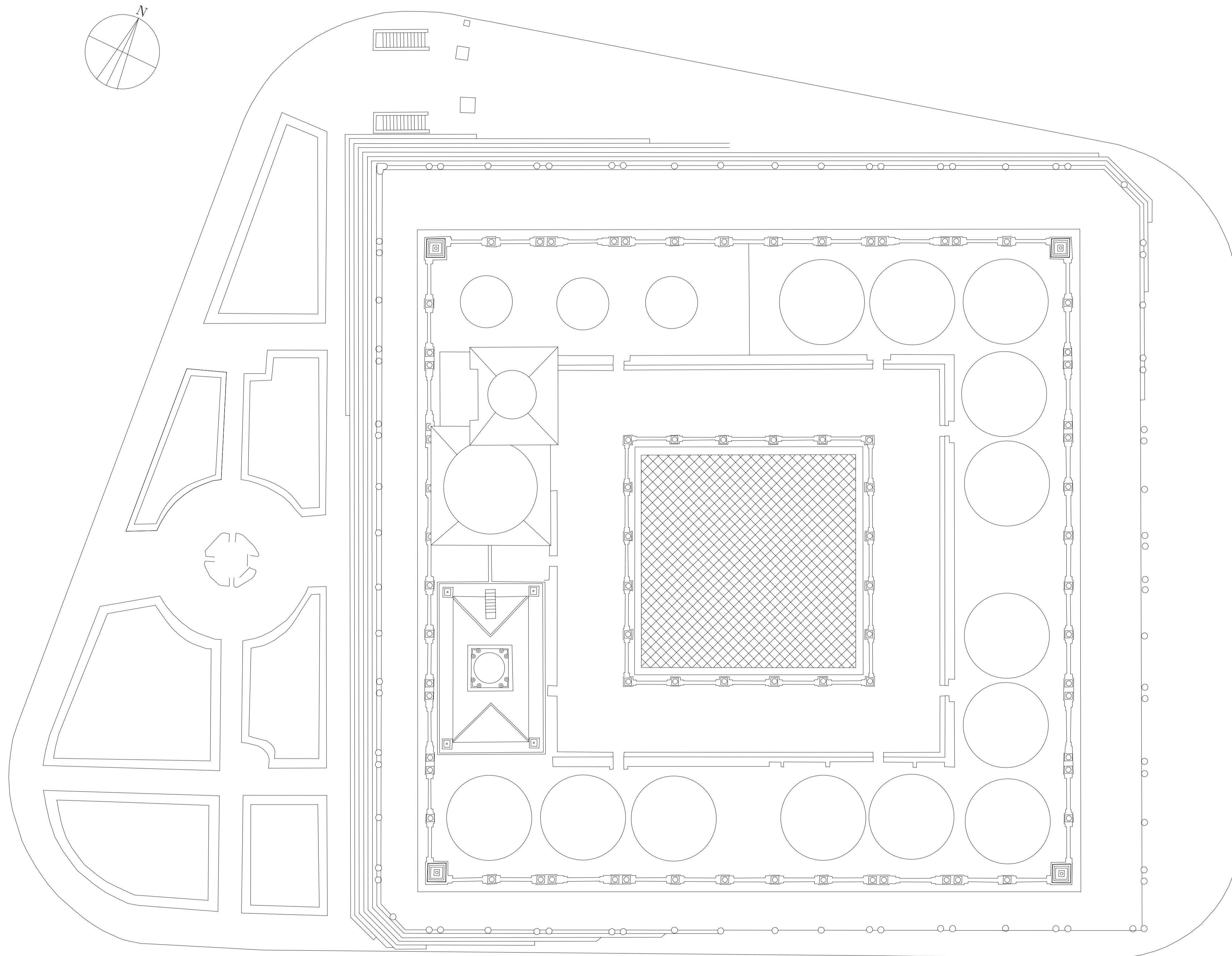
PLANTA DE CUBIERTAS
