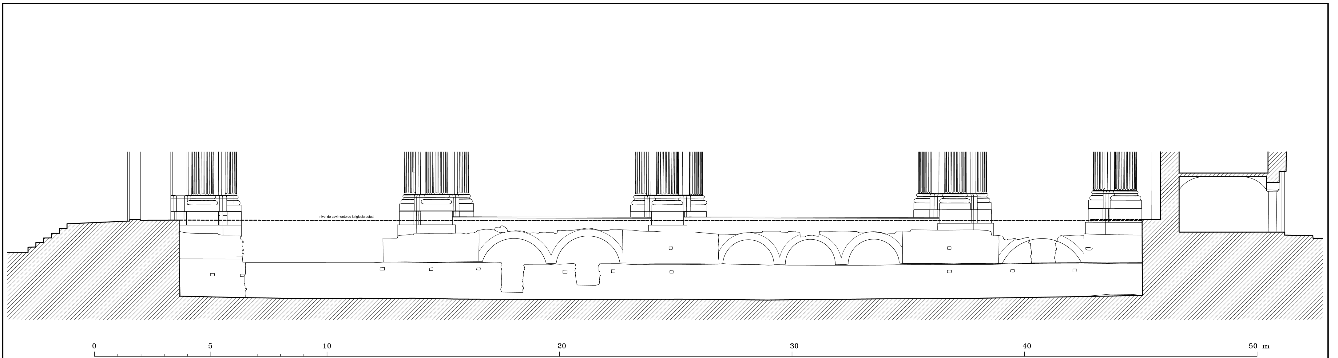
IGLESIA COLEGIAL DEL SALVADOR. SEVILLA. SECCIÓN DE LA CRIPTA POR LA NAVE DEL EVANGELIO ESCUELA DE ESTUDIOS ÁRABES. CSIC. Antonio Almagro /arquitecto. Septiembre 2004.
