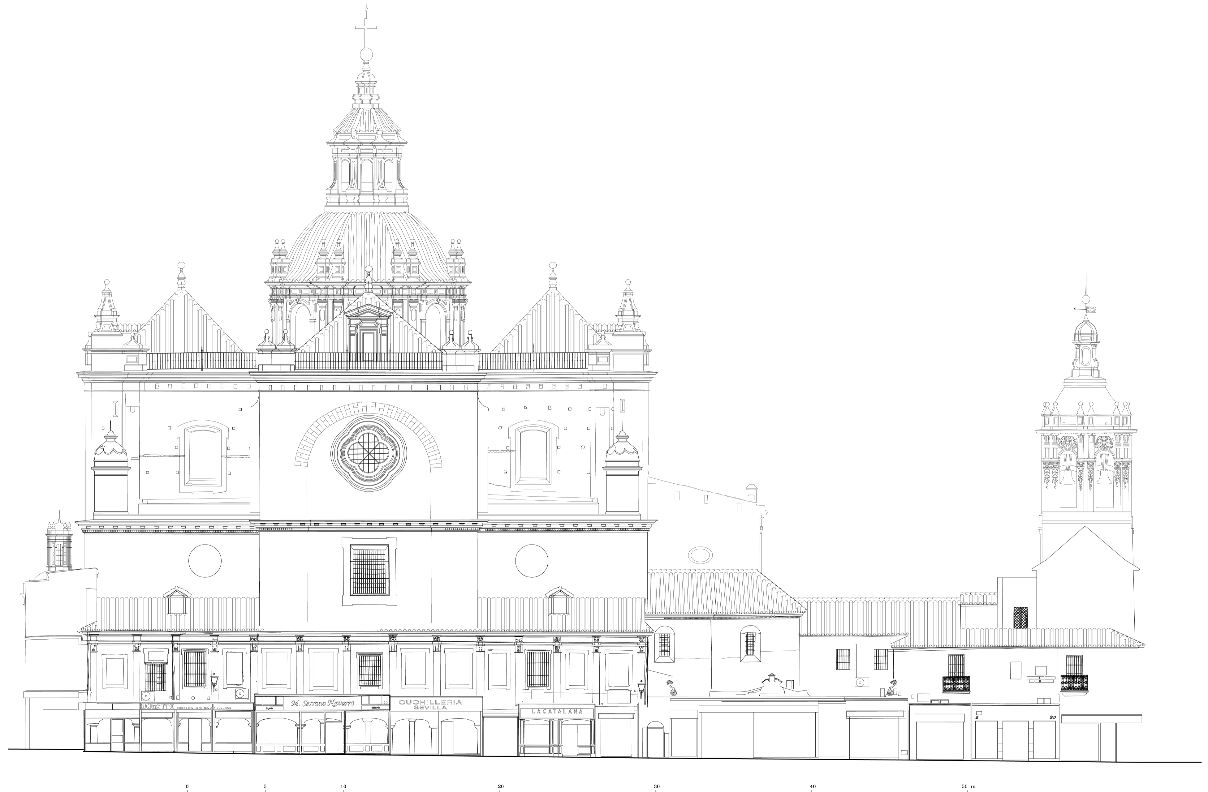
IGLESIA COLEGIAL DEL SALVADOR. SEVILLA. ALZADO ESTE
