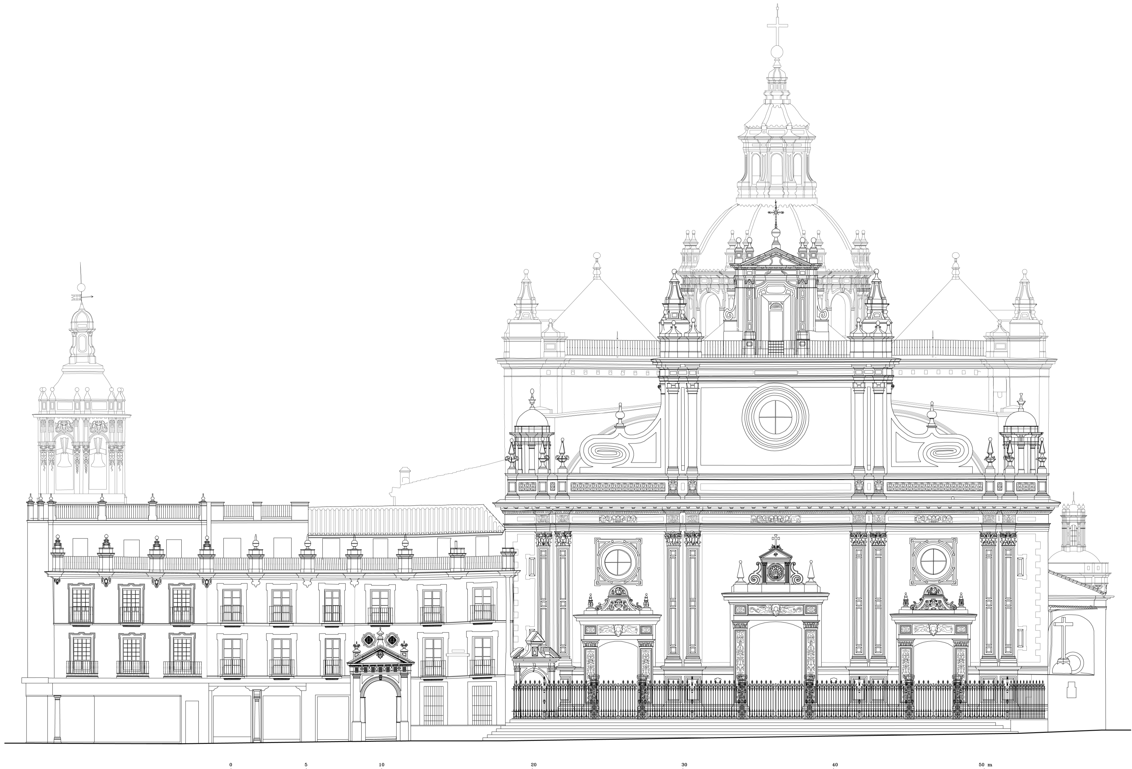
IGLESIA COLEGIAL DEL SALVADOR. SEVILLA. ALZADO PRINCIPAL ESCUELA DE ESTUDIOS ÁRABES. CSIC. Antonio Almagro /arquitecto. Septiembre 2004.
