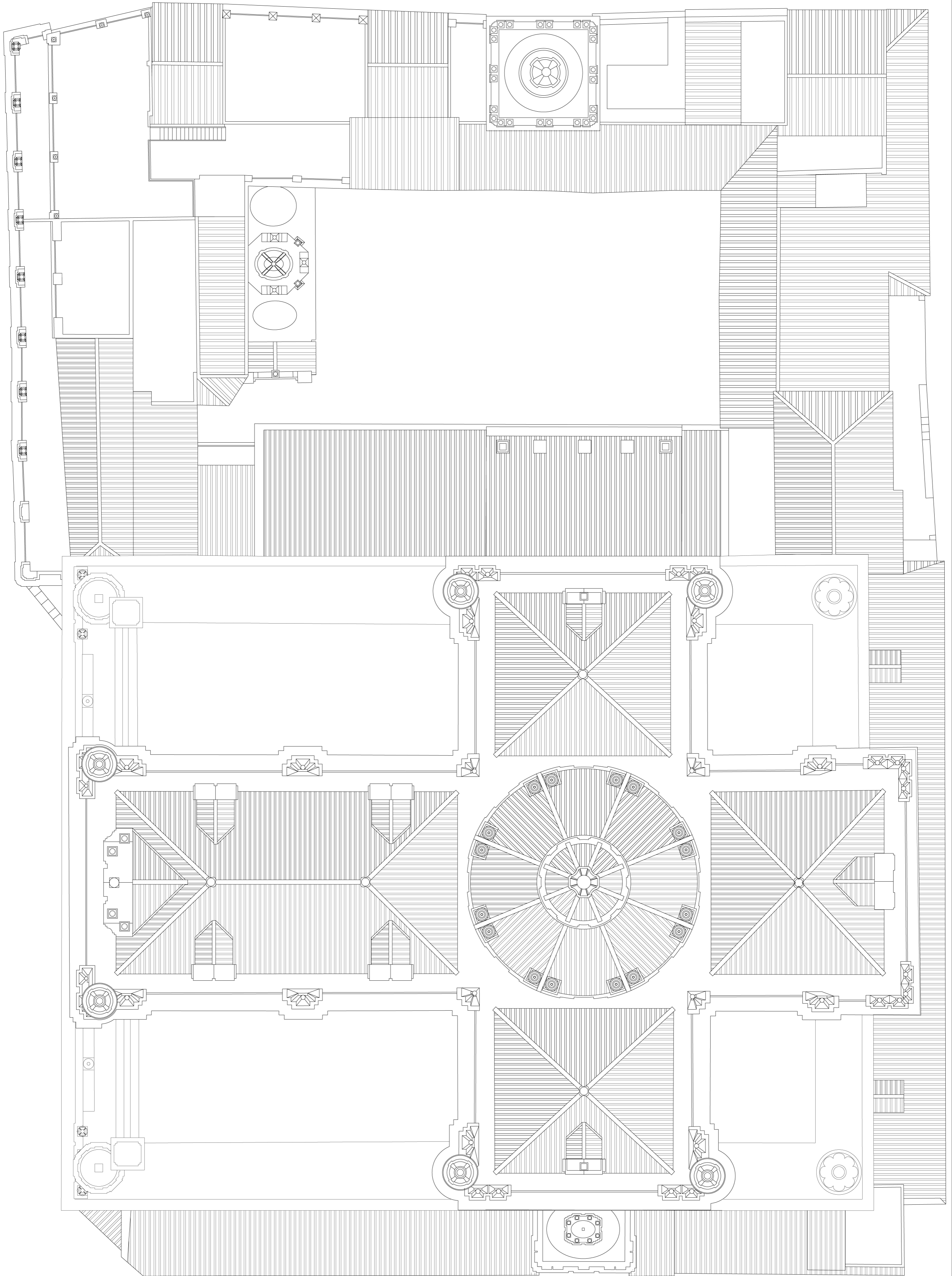
IGLESIA COLEGIAL DEL SALVADOR. SEVILLA. PLANTA DE CUBIERTAS ESCUELA DE ESTUDIOS ÁRABES. CSIC. Antonio Almagro /arq. Septiembre 2005.
