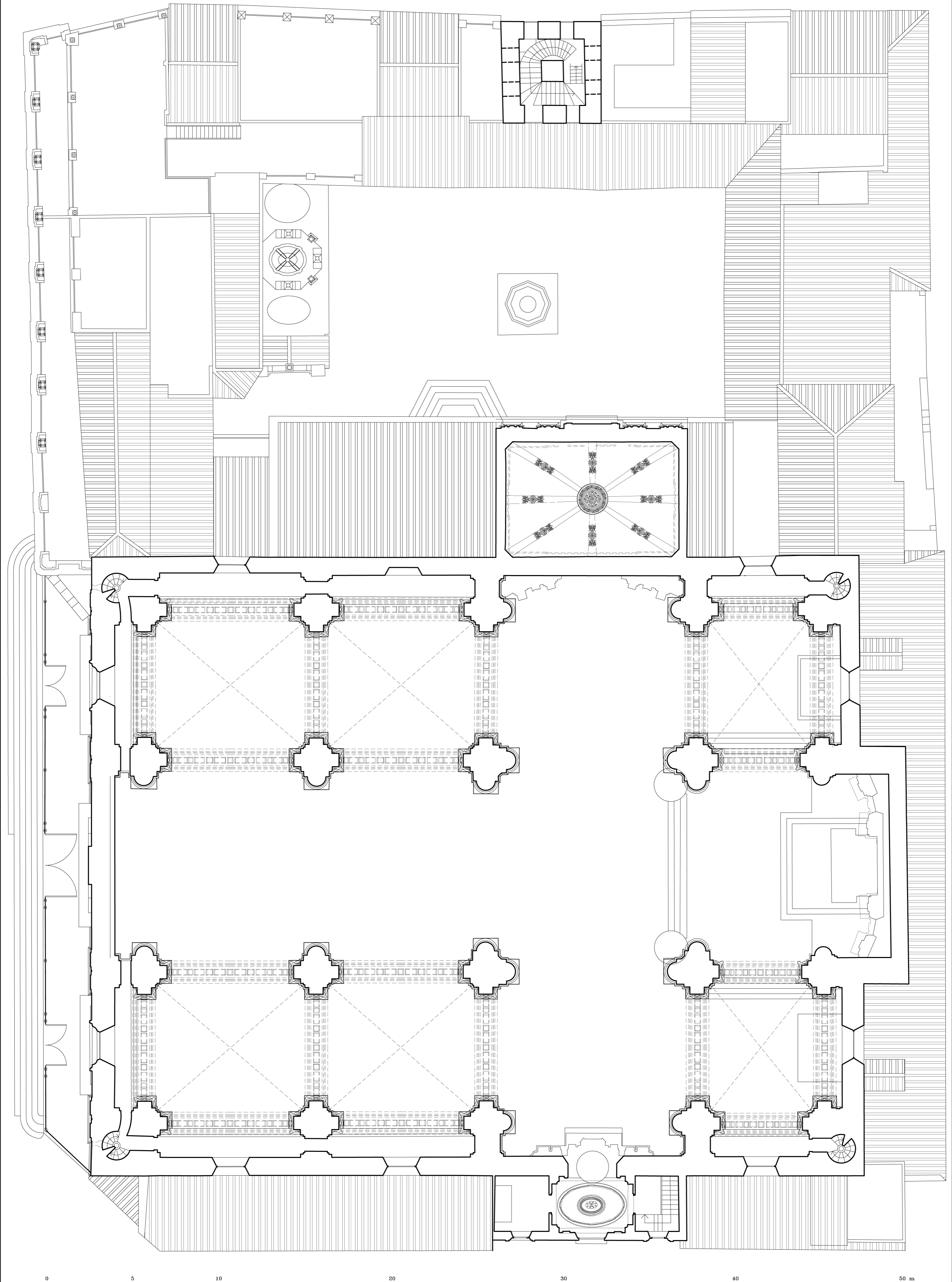
IGLESIA COLEGIAL DEL SALVADOR. SEVILLA. PLANTA A NIVEL DE LAS TRIBUNAS ESCUELA DE ESTUDIOS ÁRABES. CSIC. Antonio Almagro /arq. Septiembre 2005.
