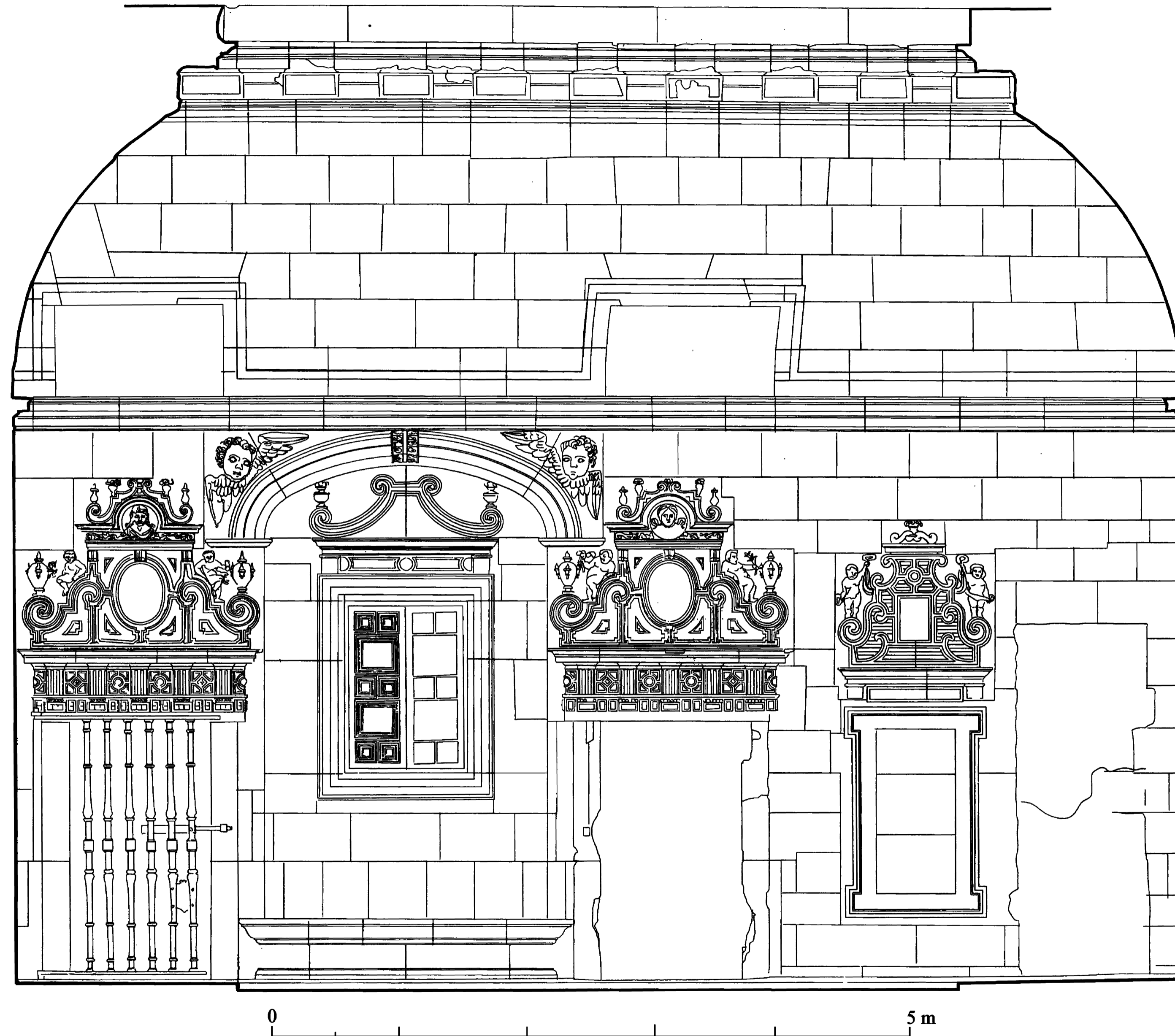
CATEDRAL METROPOLITANA DE SEVILLA. SECCION DEL PATIO DEL MARISCAL (CABILDO). GABINETE DE FOTOGAMETRIA DEL I.C.R.B.C., A.ALMAGRO /arq.
