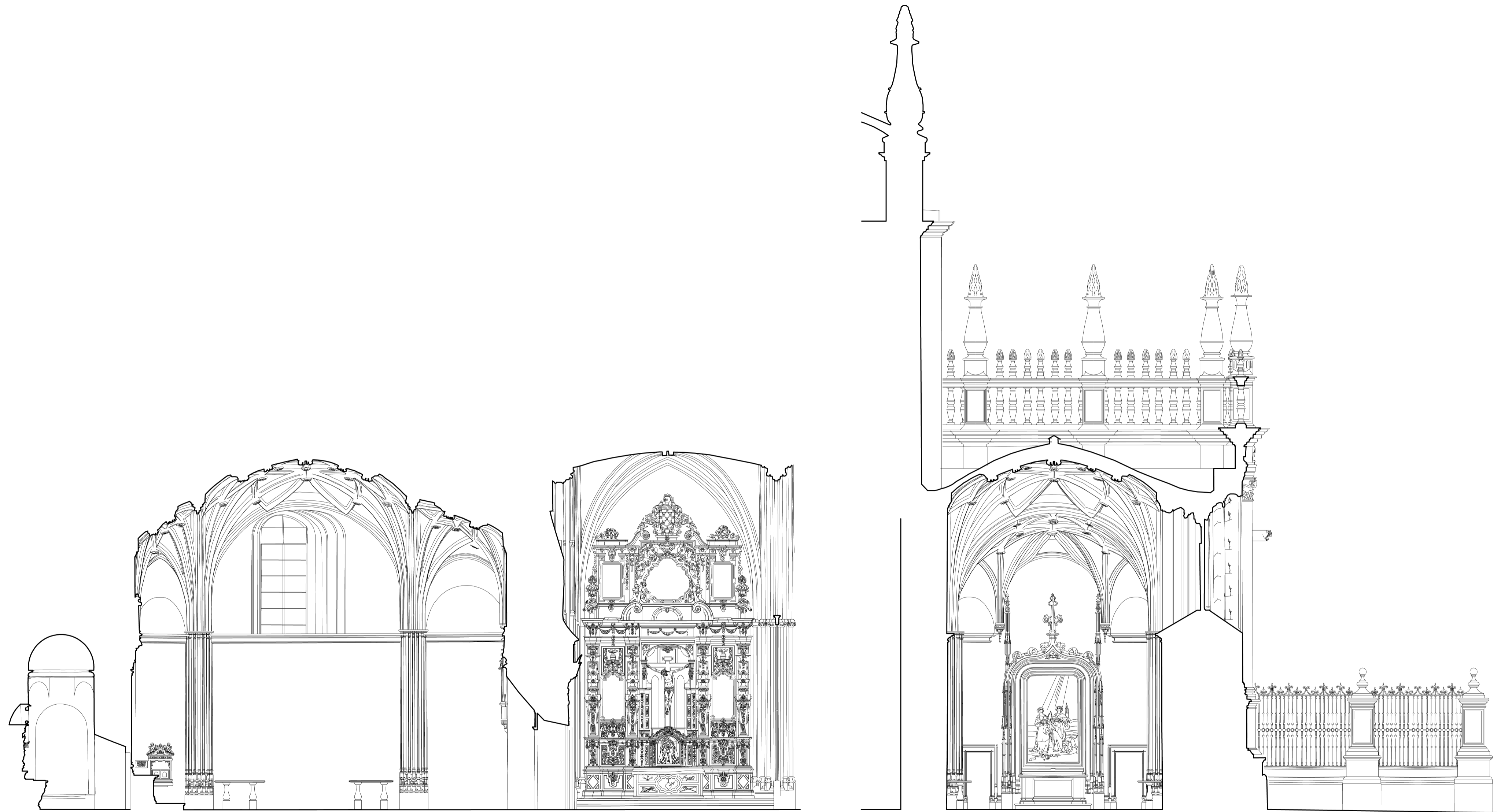
SECCIÓN LONGITUDINAL DE LA SACRISTÍA DE LOS CALICES Y CAPILLA DE LOS DOLORES
