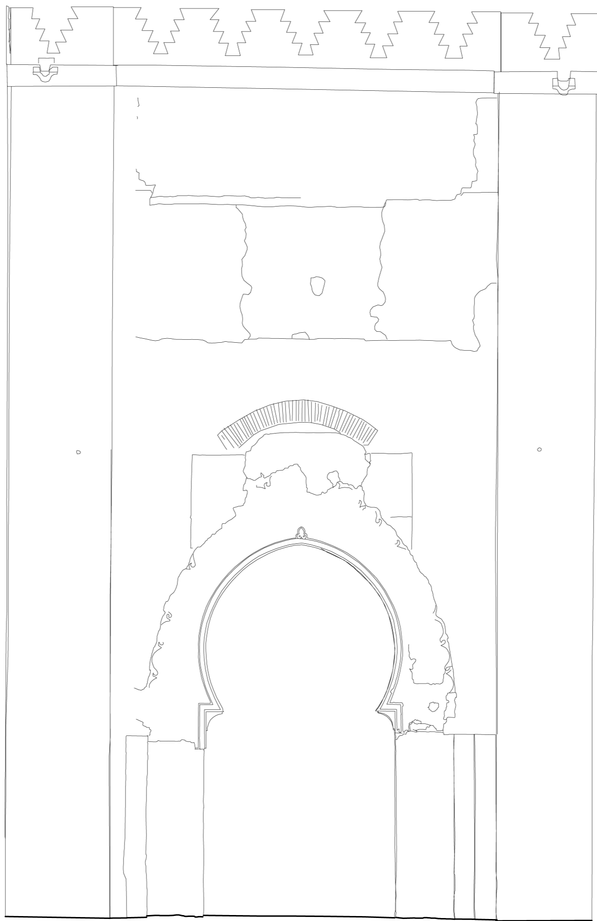
ALZADO
