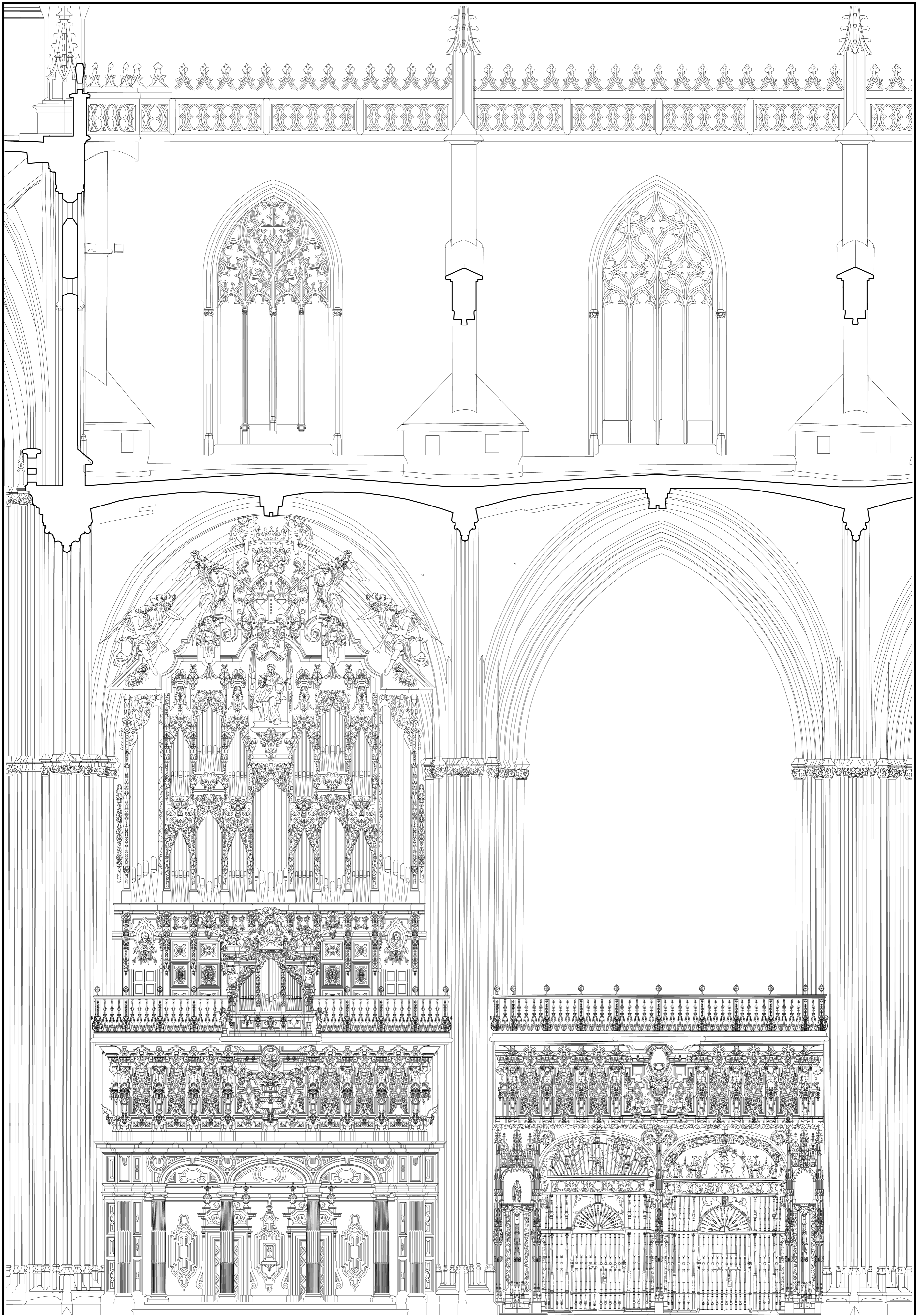
CATEDRAL METROPOLITANA DE SEVILLA. ALZADO NORTE DEL EXTERIOR DEL CORO Y EL ÓRGANO.
