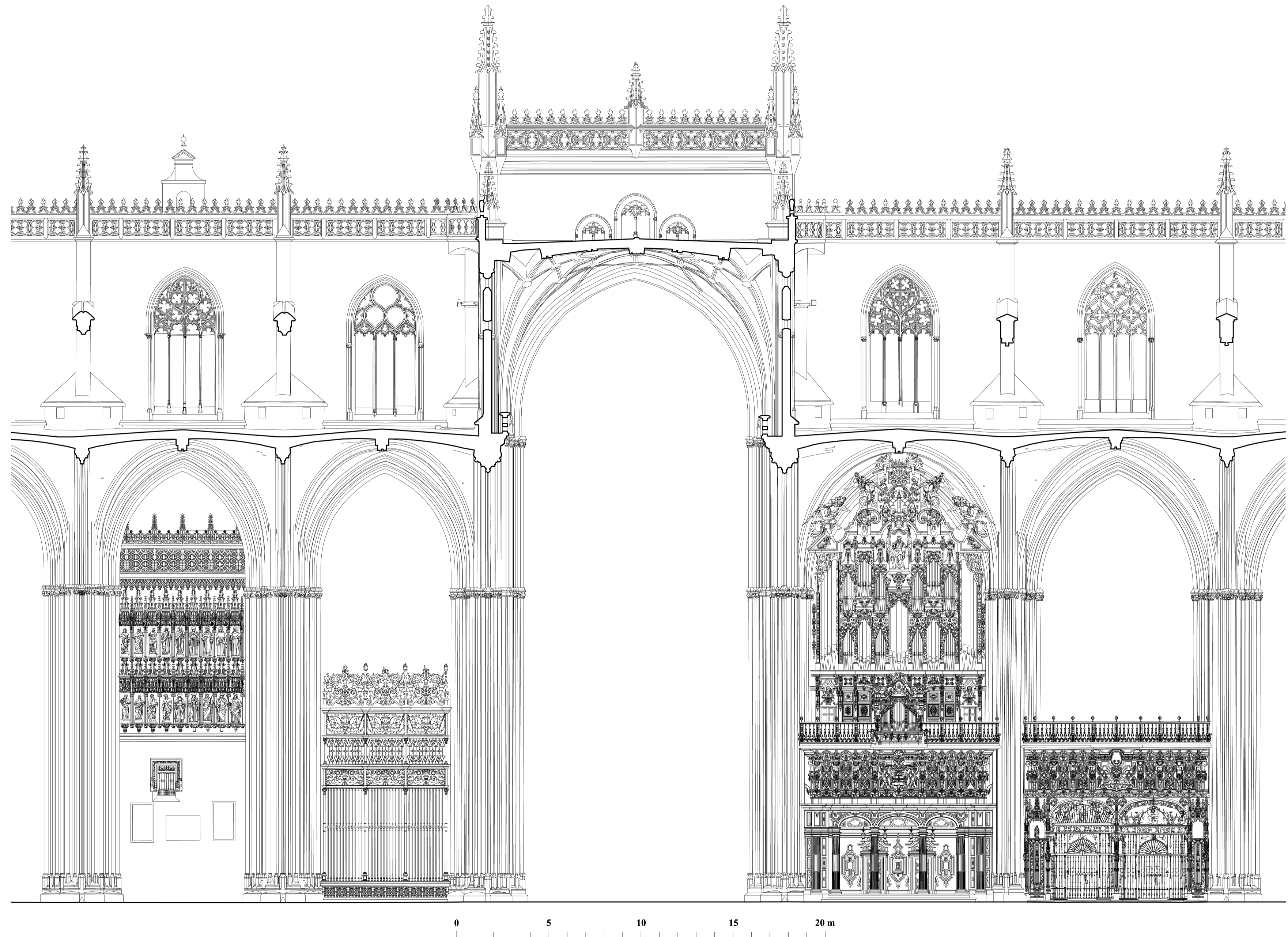
CATEDRAL METROPOLITANA DE SEVILLA. ALZADO NORTE DEL CORO Y LA CAPILLA MAYOR. ESCUELA DE ESTUDIOS ARABES, C.S.I.C. A.ALMAGRO /arq. IZUÑIGA /arq.tec.
