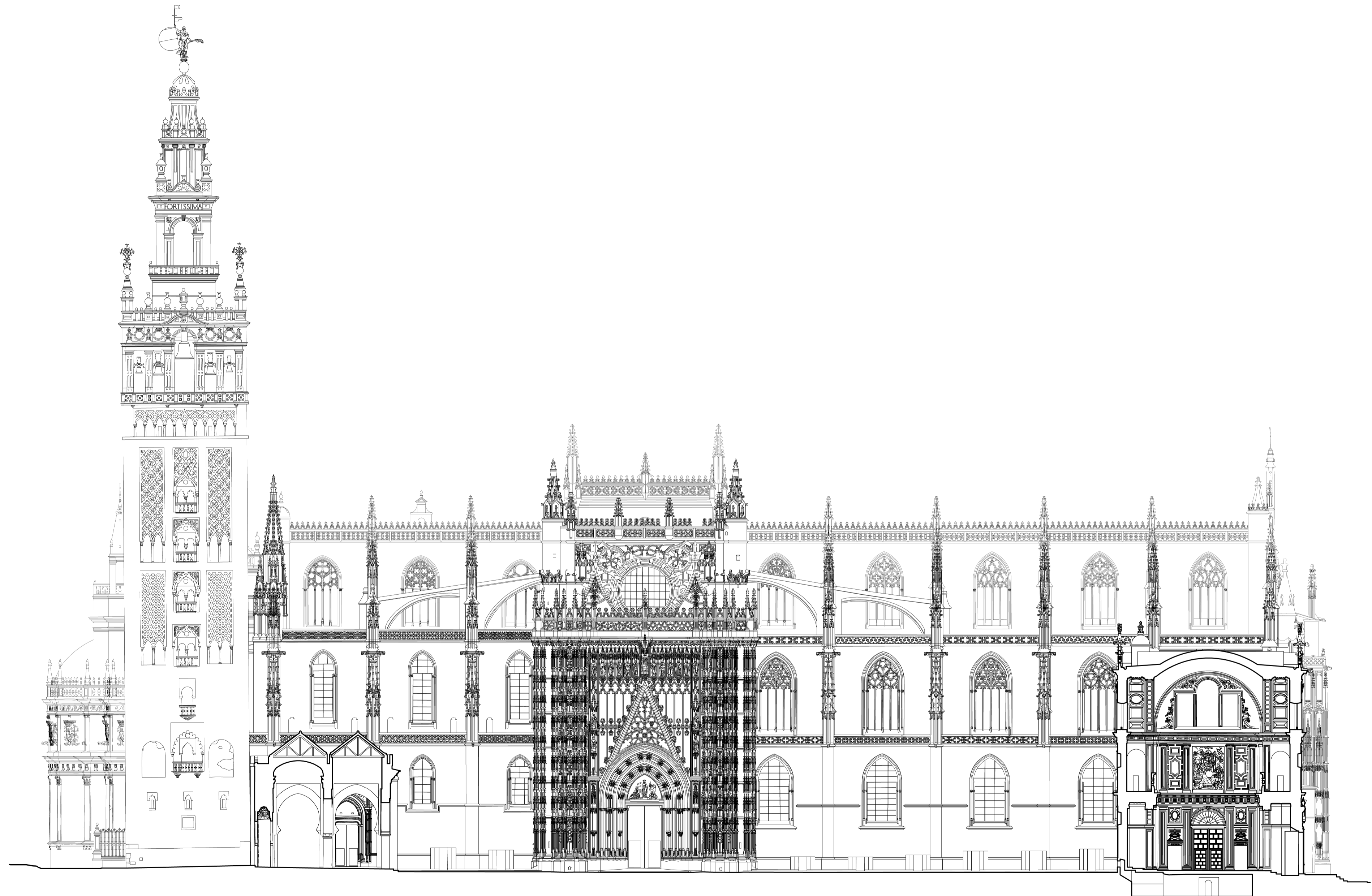
CATEDRAL METROPOLITANA DE SEVILLA. ALZADO NORTE Y SECCION DEL PATIO.
