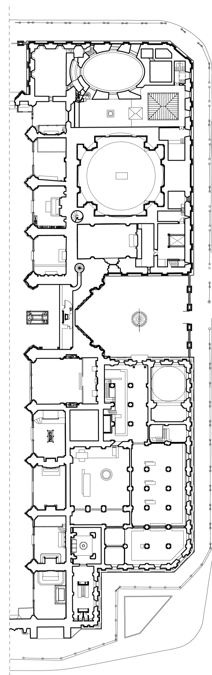
PLANTA A NIVEL DE LAS ENTREPLANTAS DE LA ZONA DEL CABLEJO.
