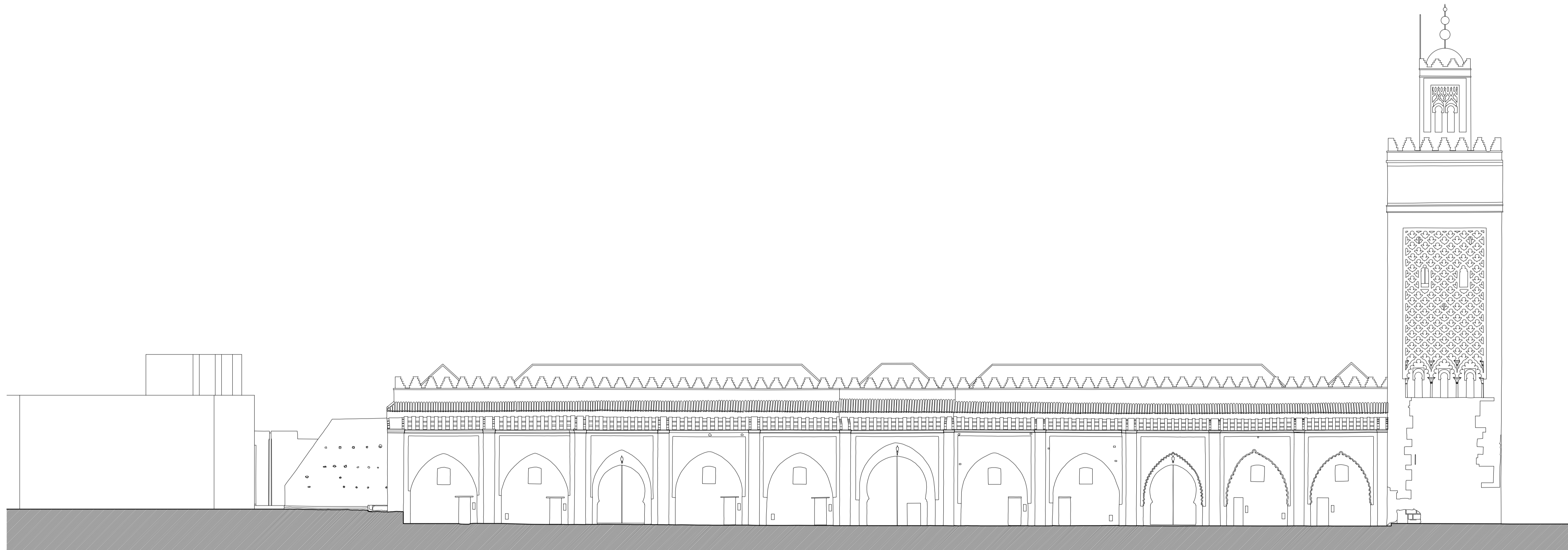
ALZADO SEPTENTRIONAL
