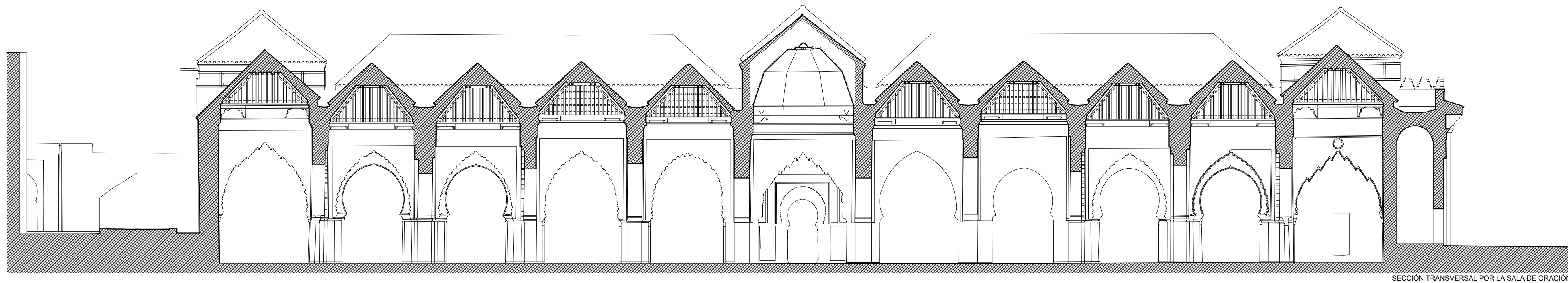
SECCIÓN TRANSVERSAL POR LA SALA DE ORACIÓN
