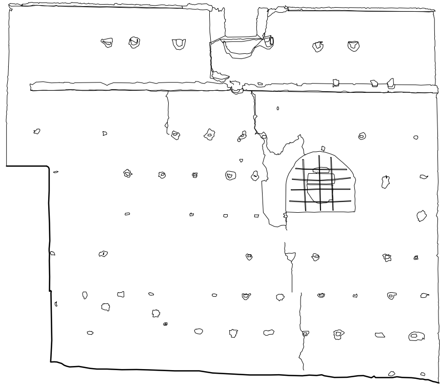
AGDAL DE MARRAKECH. BASTIÓN SUROESTE. ALZADO NORTE. ANTONIO ALMAGRO, arquitecto, JULIO 2013
