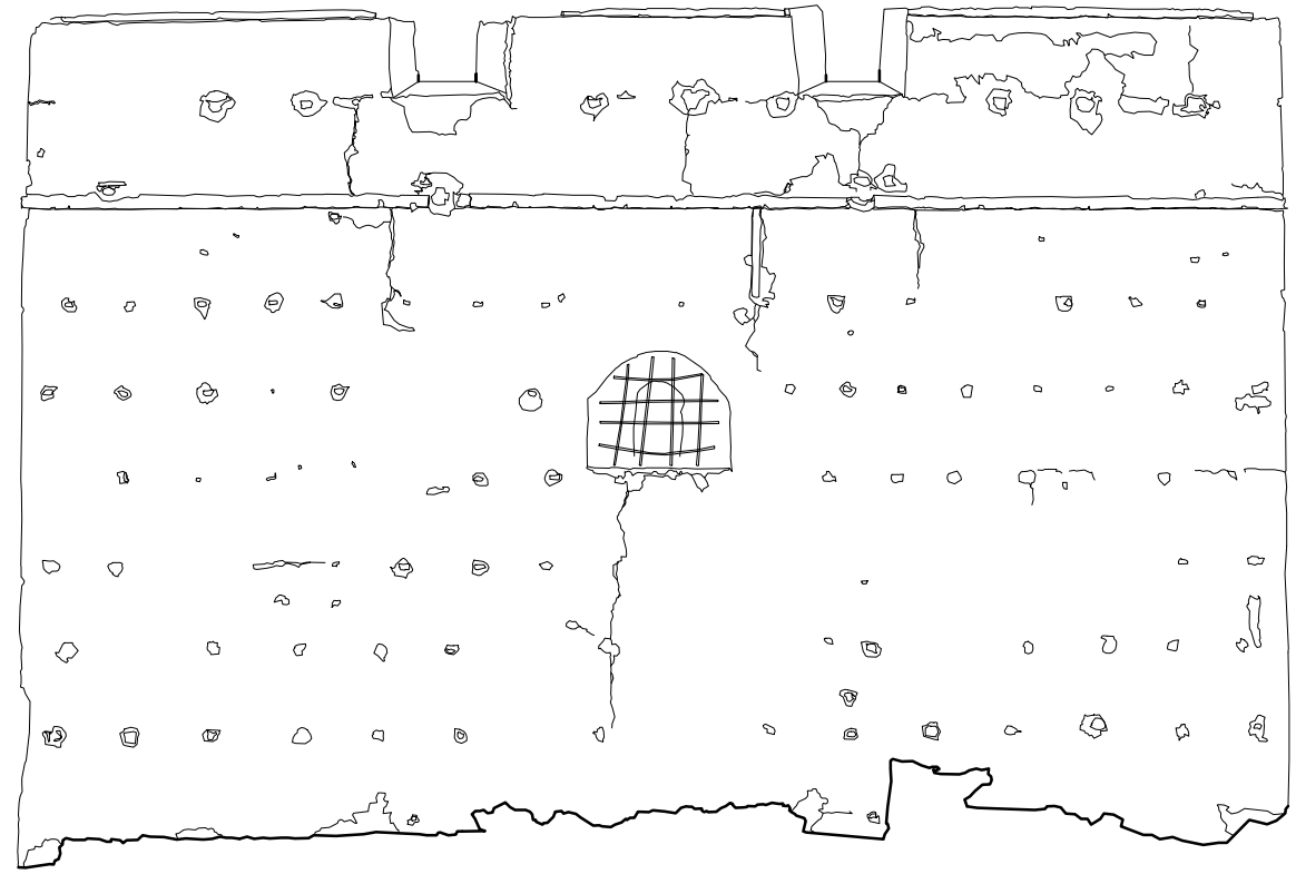
AGDAL DE MARRAKECH. BASTIÓN SUROESTE. ALZADO SUR. ANTONIO ALMAGRO, arquitecto, JULIO 2013
