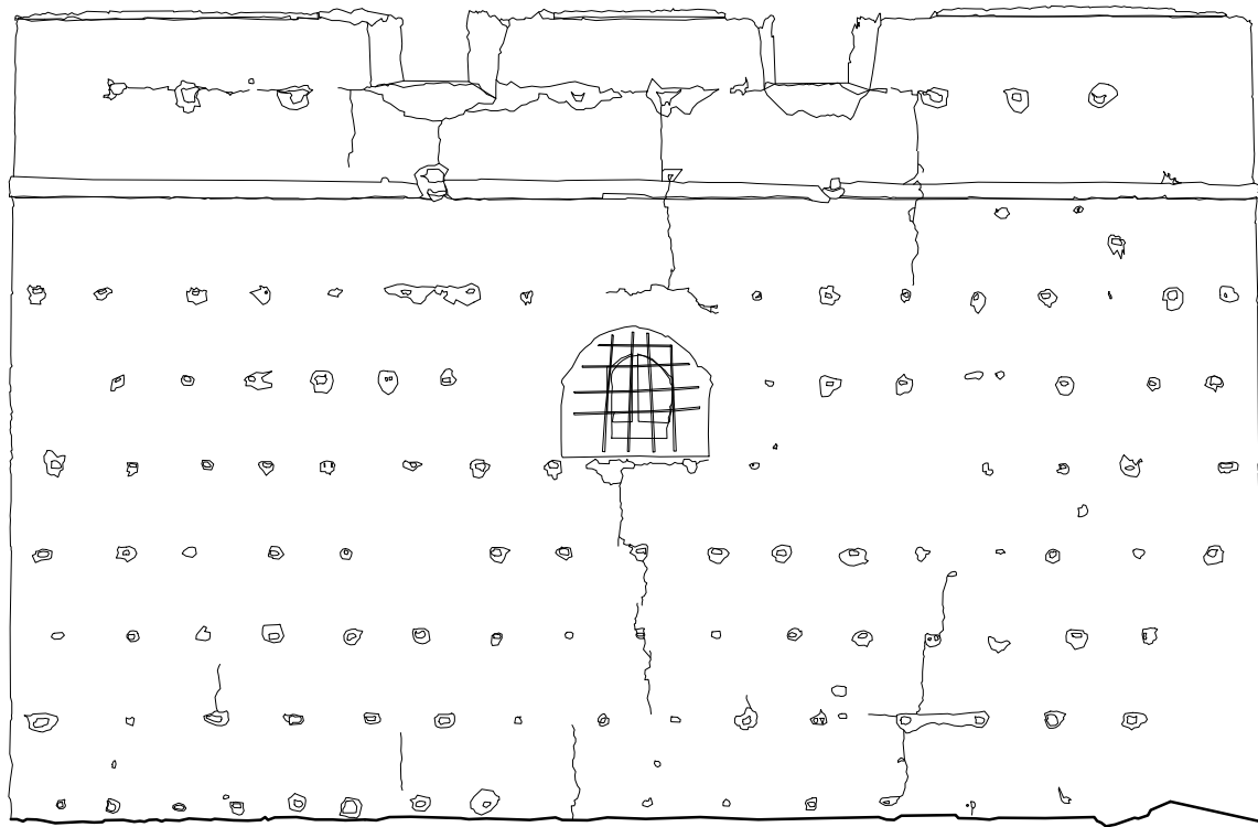
AGDAL DE MARRAKECH. BASTIÓN SUROESTE. ALZADO OESTE. ANTONIO ALMAGRO, arquitecto, JULIO 2013
