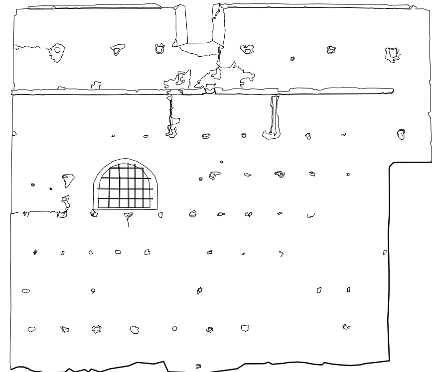
AGDAL DE MARRAKECH. BASTIÓN SUROESTE. ALZADO ESTE. ANTONIO ALMAGRO, arquitecto, JULIO 2013
