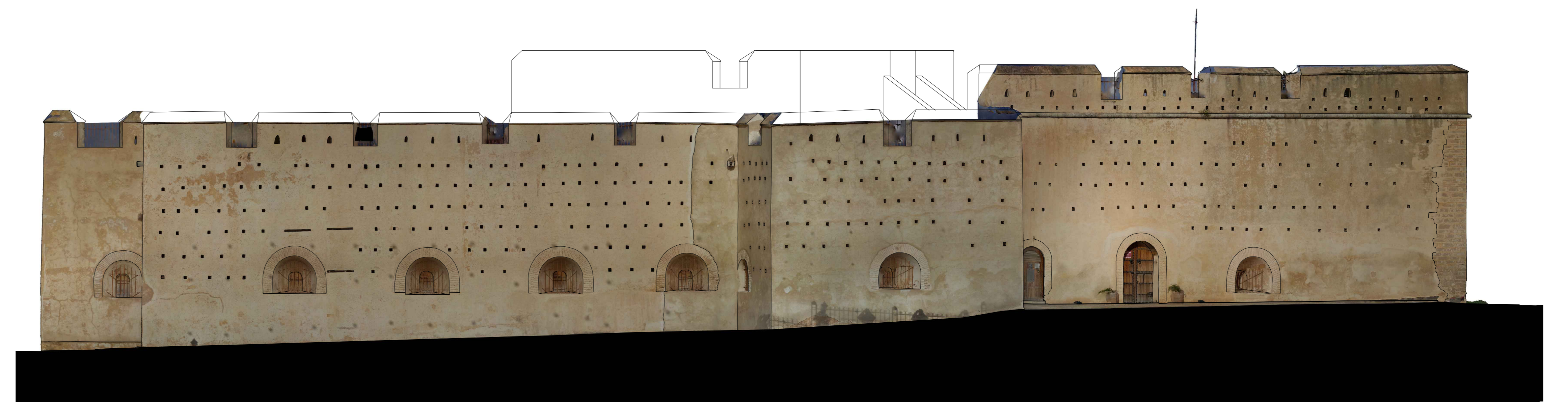
ALZADO OESTE
