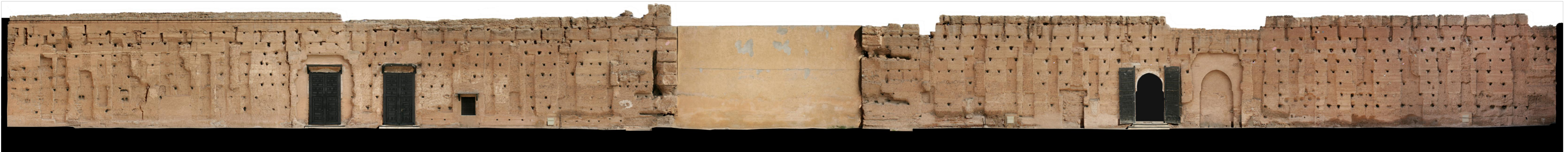
PALAIS AL-BADI' DE MARRAKECH. ÉLEVATION EST DE LA COUR. A. ALMAGRO / arch. Escuela de Estudios Árabes, CSIC. 2005-2015
