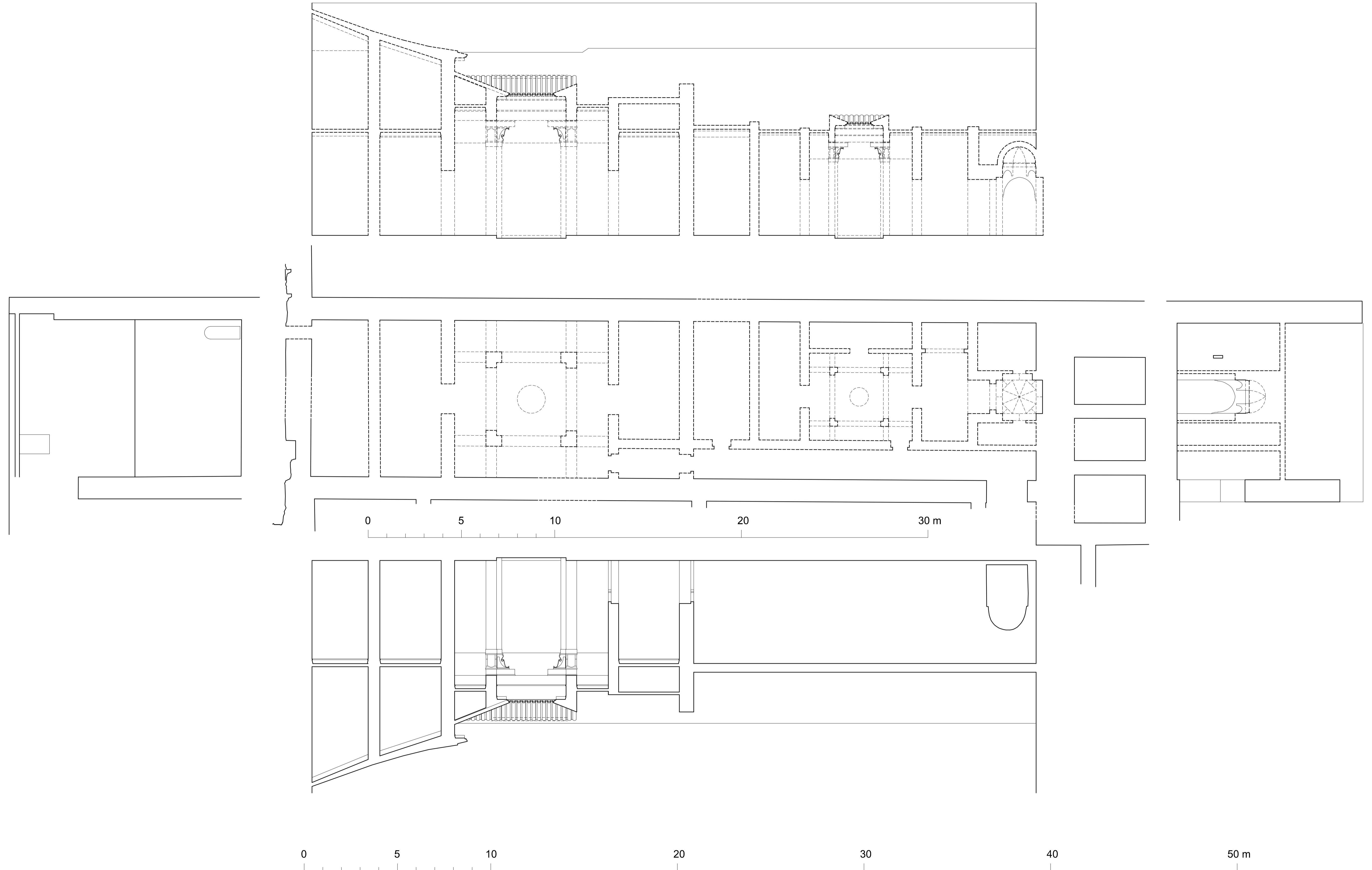
PALAIS AL-BADI' DE MARRAKECH. ZONE RÉSIDENTIELLE DU COTÉ NORD-EST
