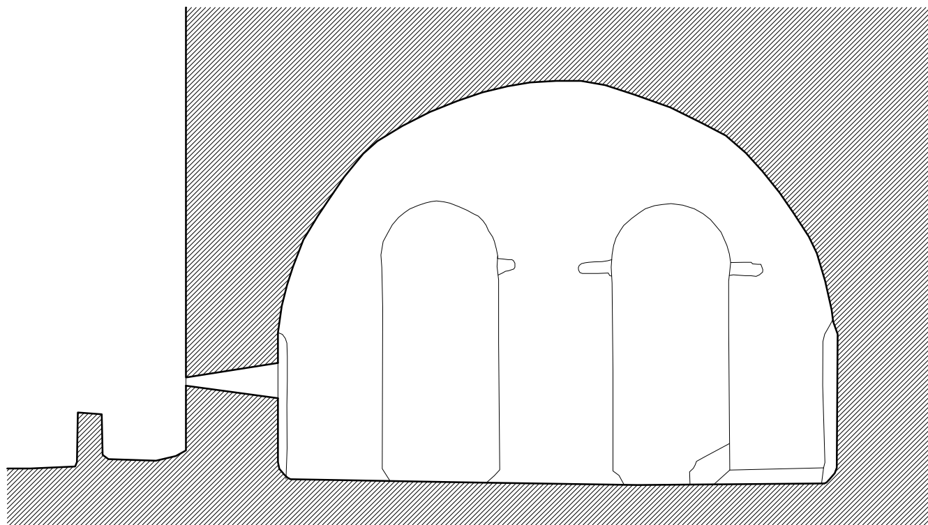
SECCIÓN DEL ALJIBE
