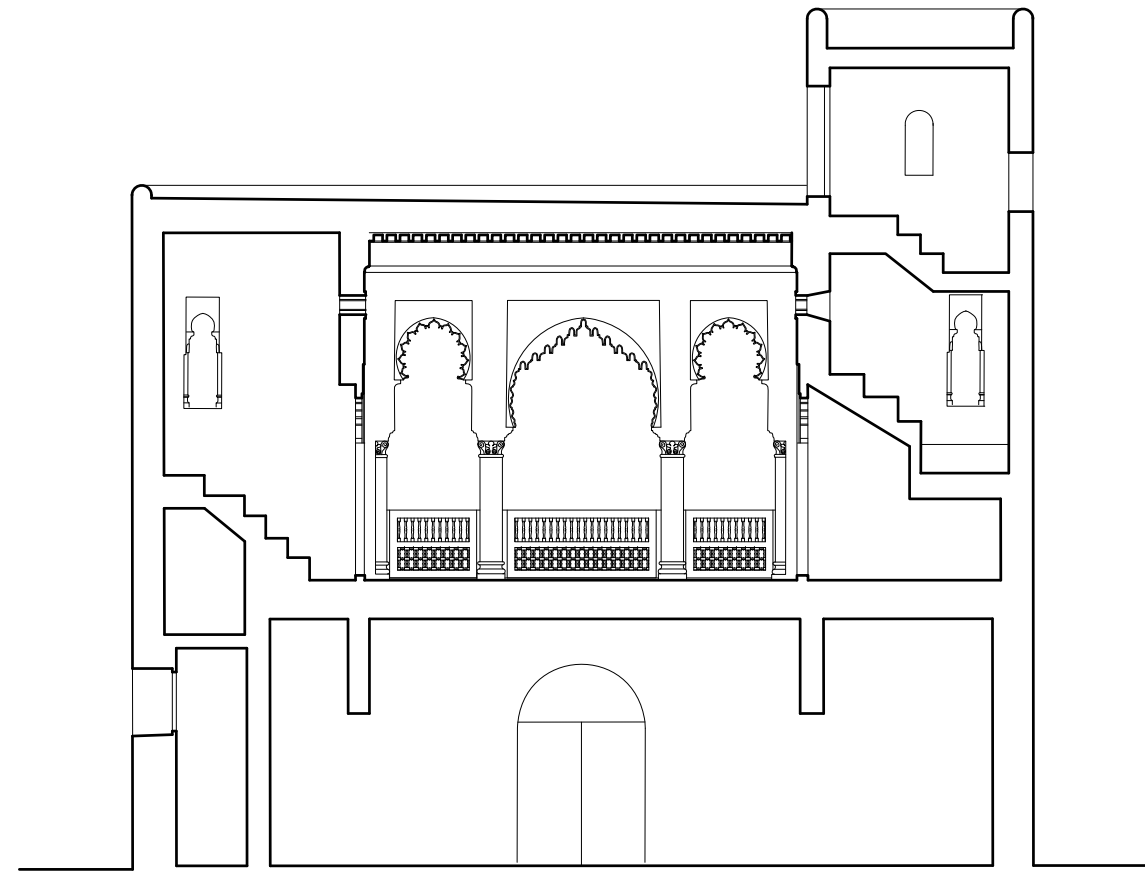
SECTION A-A
