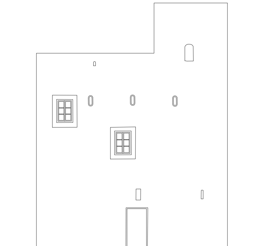
ÉLÉVATION EST
