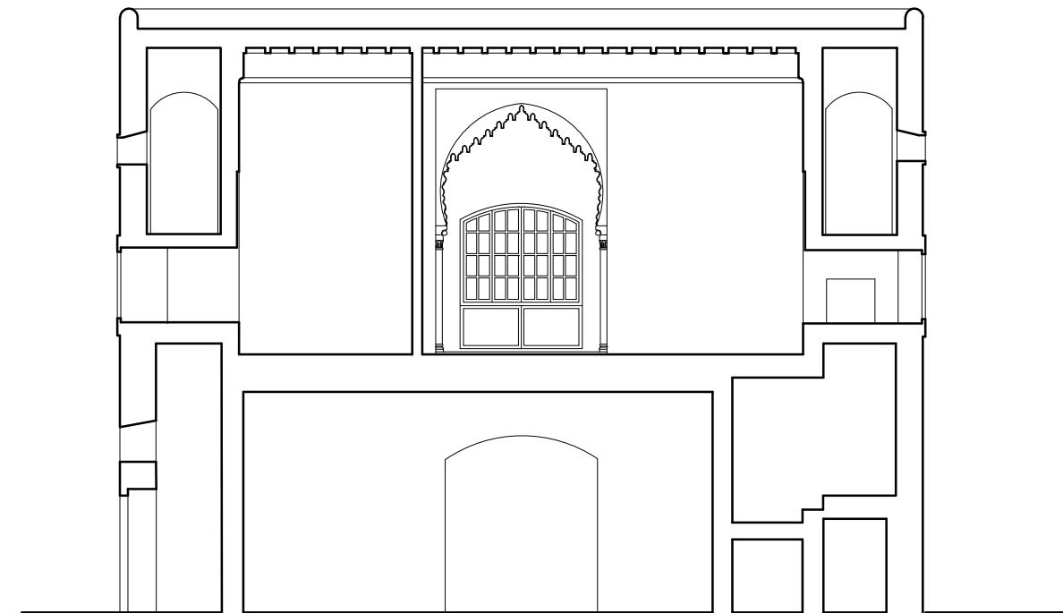
SECTION D-D
