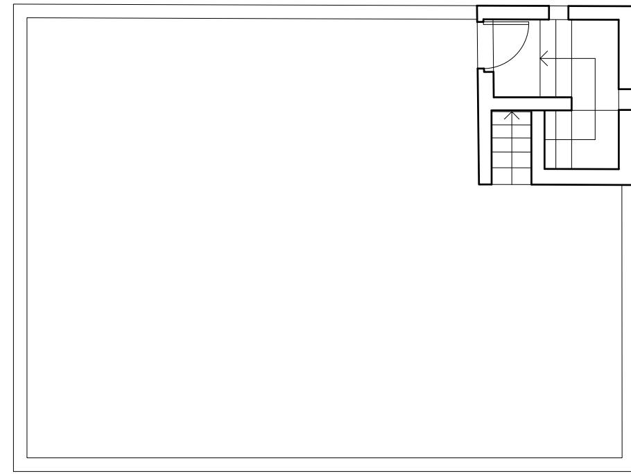
PLAN TERRASSE
