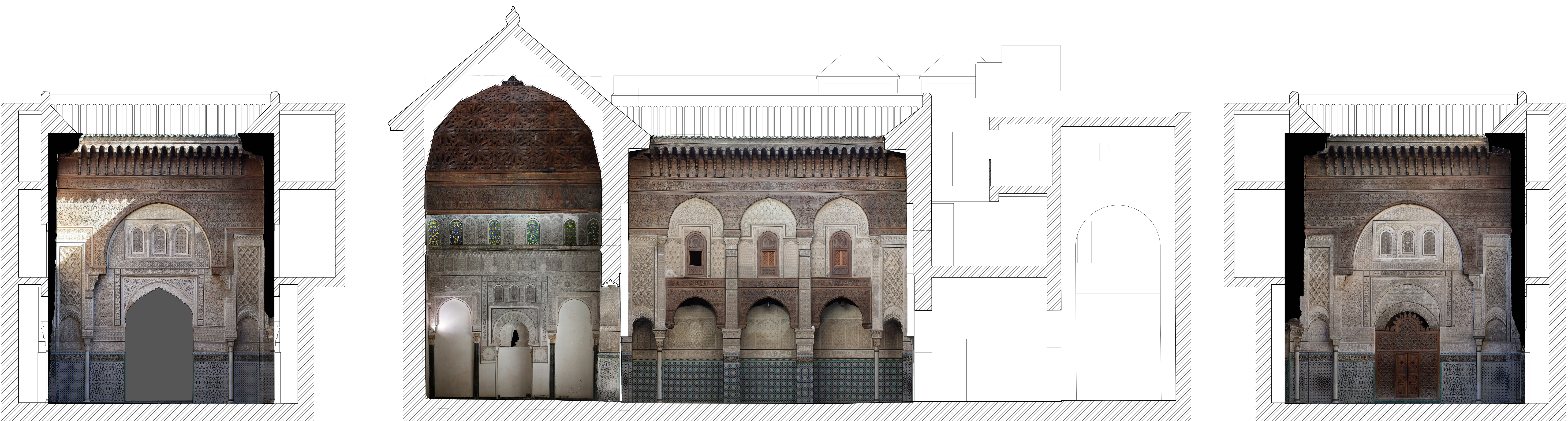
MADRASA AL-ATTARIN DE FEZ. SECCIONES A. ALMAGRO y I. ALMELA / arq. ESCUELA DE ESTUDIOS ARABES, CSIC MAYO 2017
