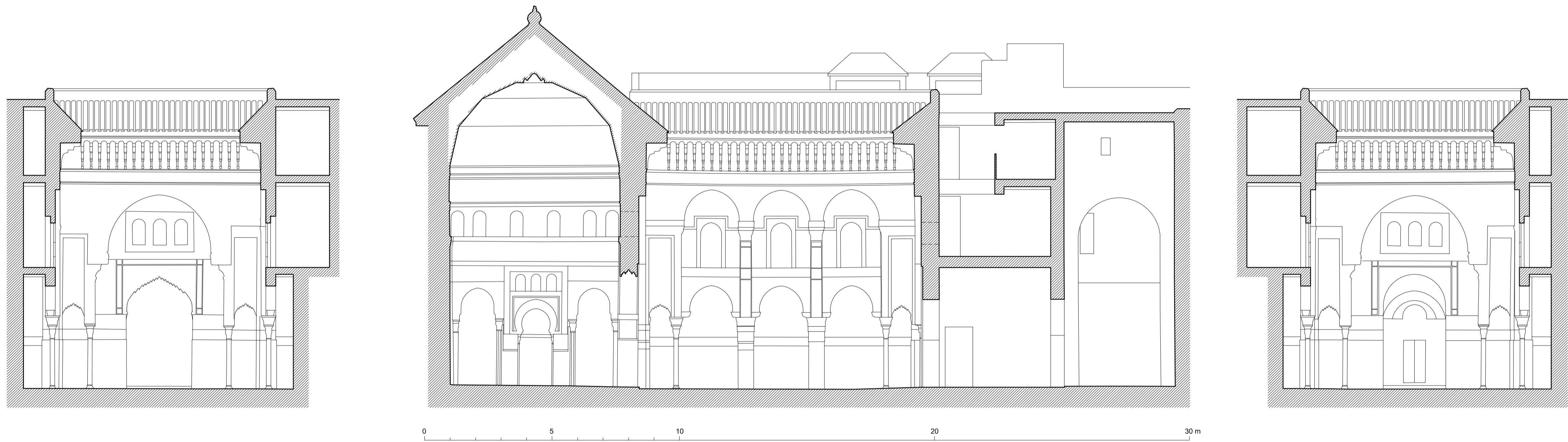
MADRASA AL-ATTARIN DE FEZ. SECCIONES A. ALMAGRO / I. ARANDA / IUL EDUCACIÓN DE ESTUDIOS BÁSICOS, S.L. 1997-2017
