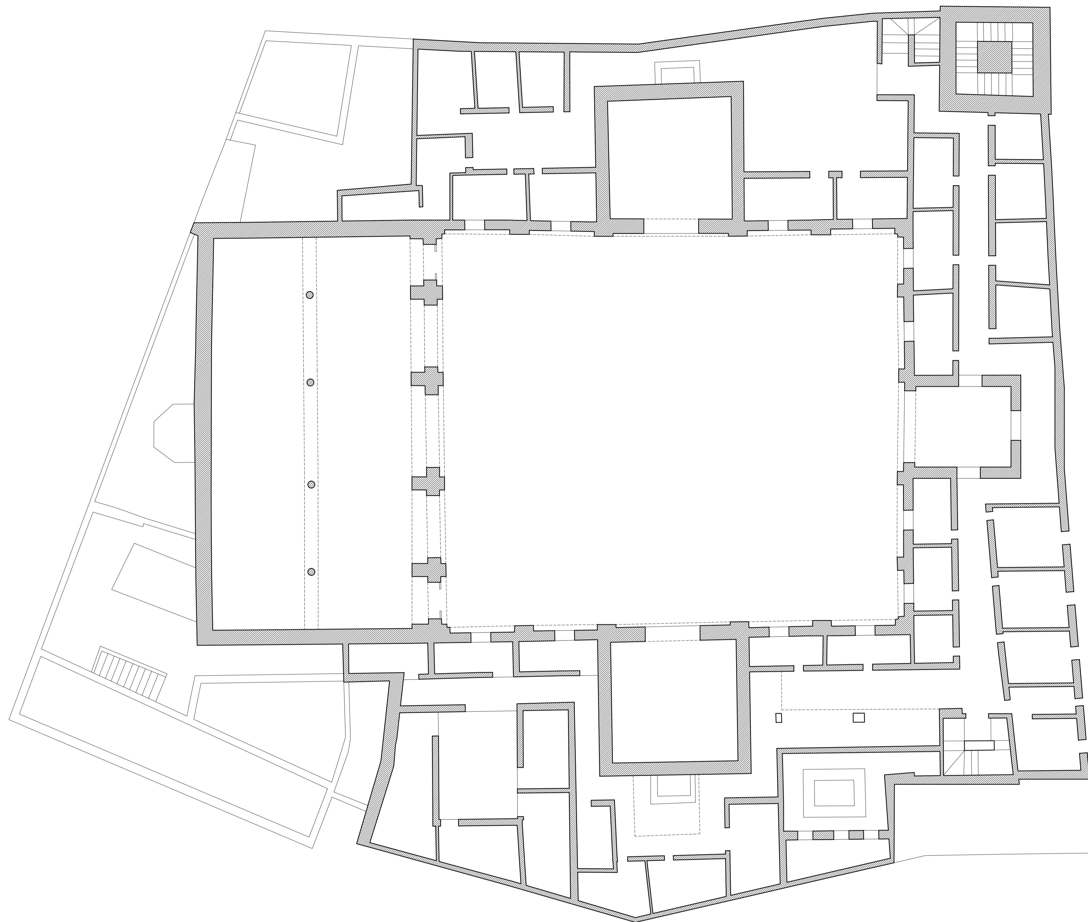
MADRASA BU INANIA DE FEZ. PLANTA ALTA A. ALMAGRO y I. ALMELA / arq. ESCUELA DE ESTUDIOS ÁRABES, CSIC MAYO 2017
